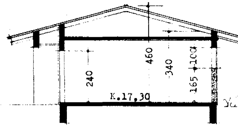
skurður B-B
