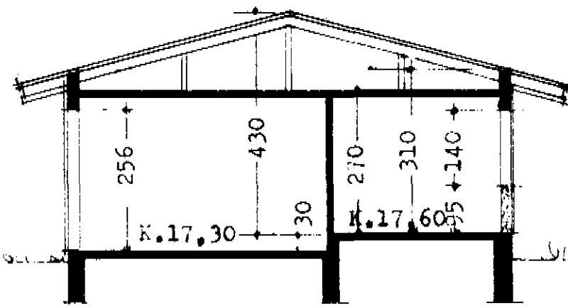
skurður A-A
