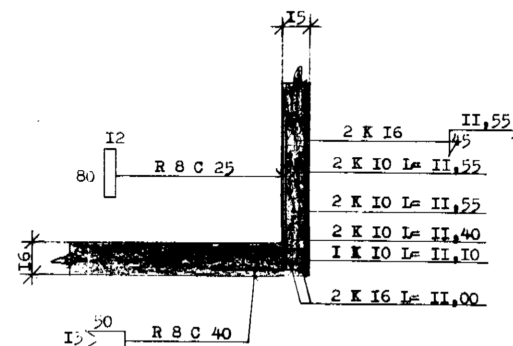
SNID G - G I:20
