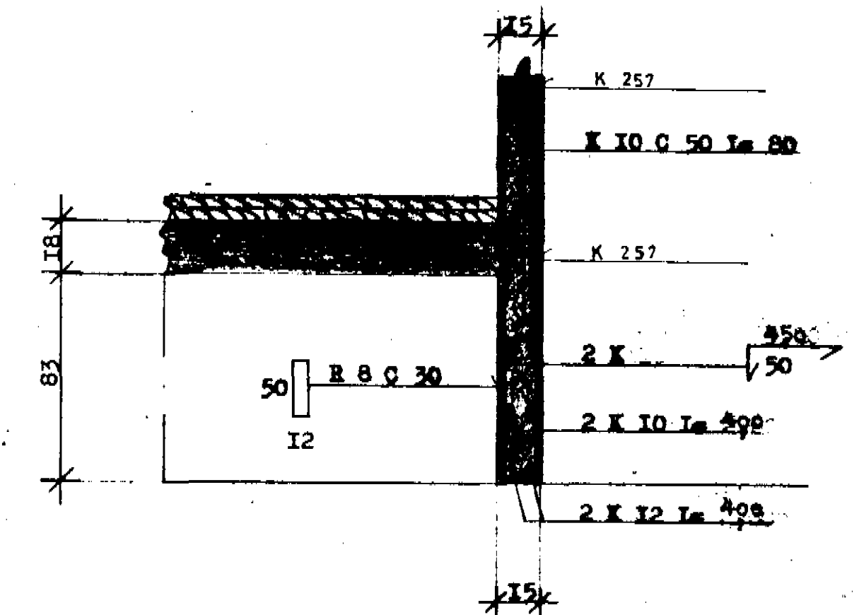
SNID H - H I:20
