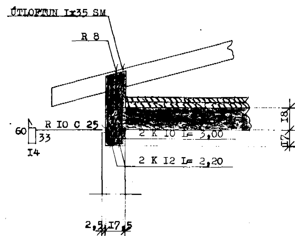
SNID F - F I:20
