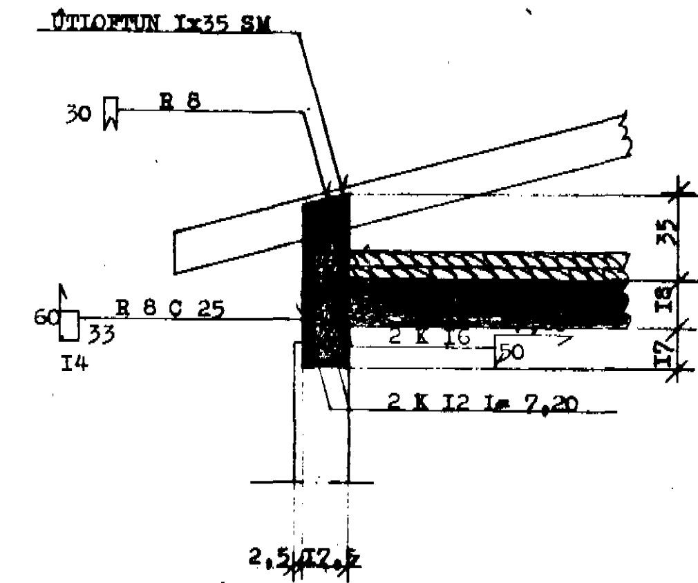
SNID D - D I:20
