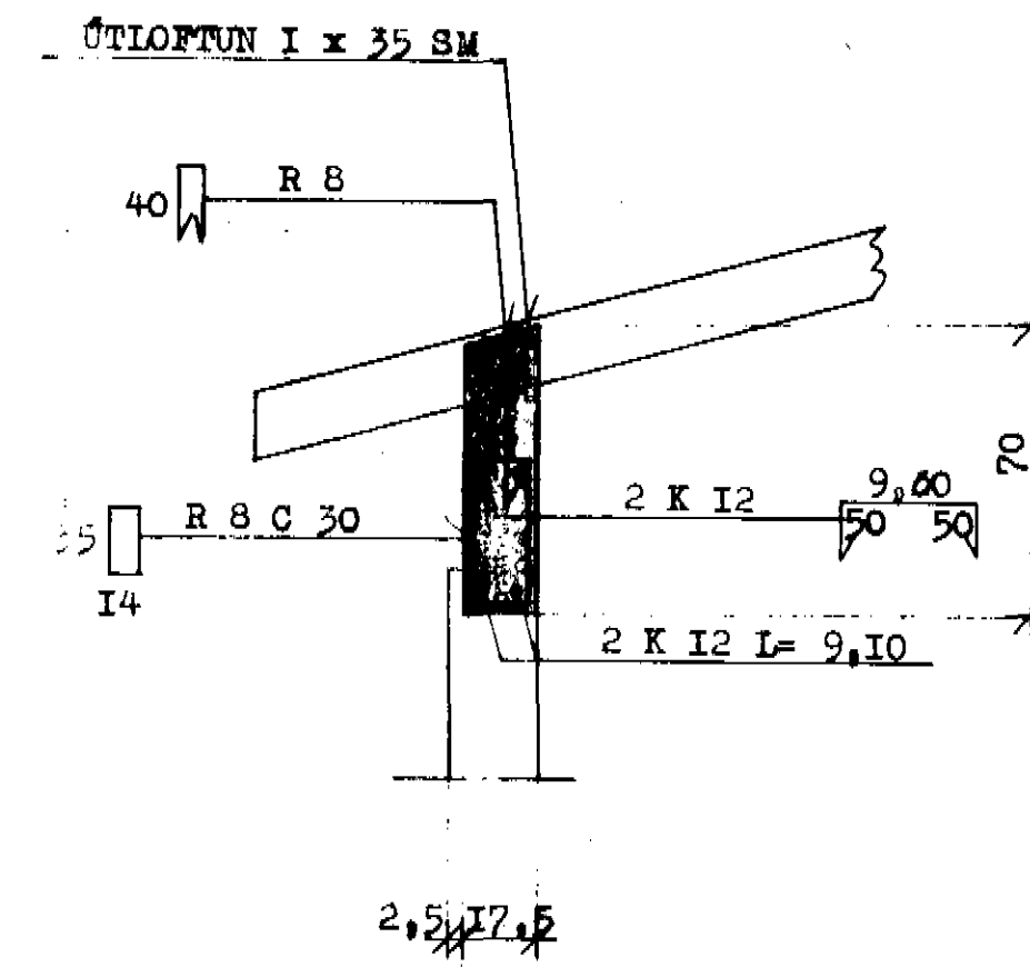
SNID C - C I:20
