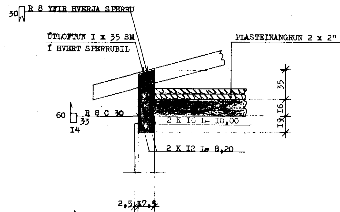
SNID A - A I:20
