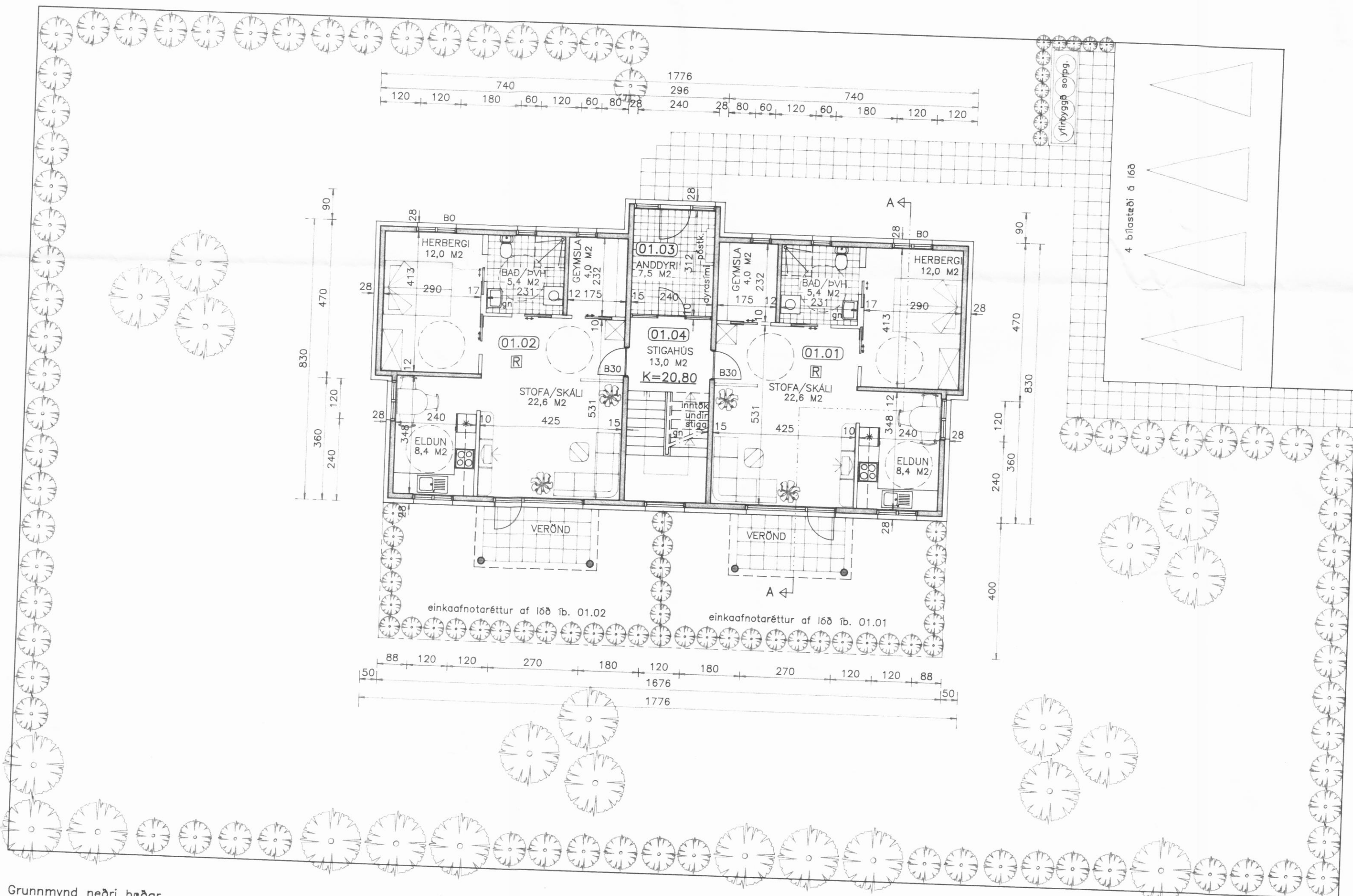
Grunnmynd neðri hæðar mkv. 1:100
