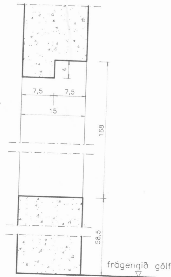
SNID 1-1 mkv. 1:5
