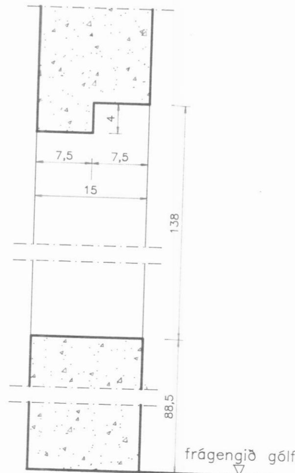
SNID 1-1 mkv. 1:5
