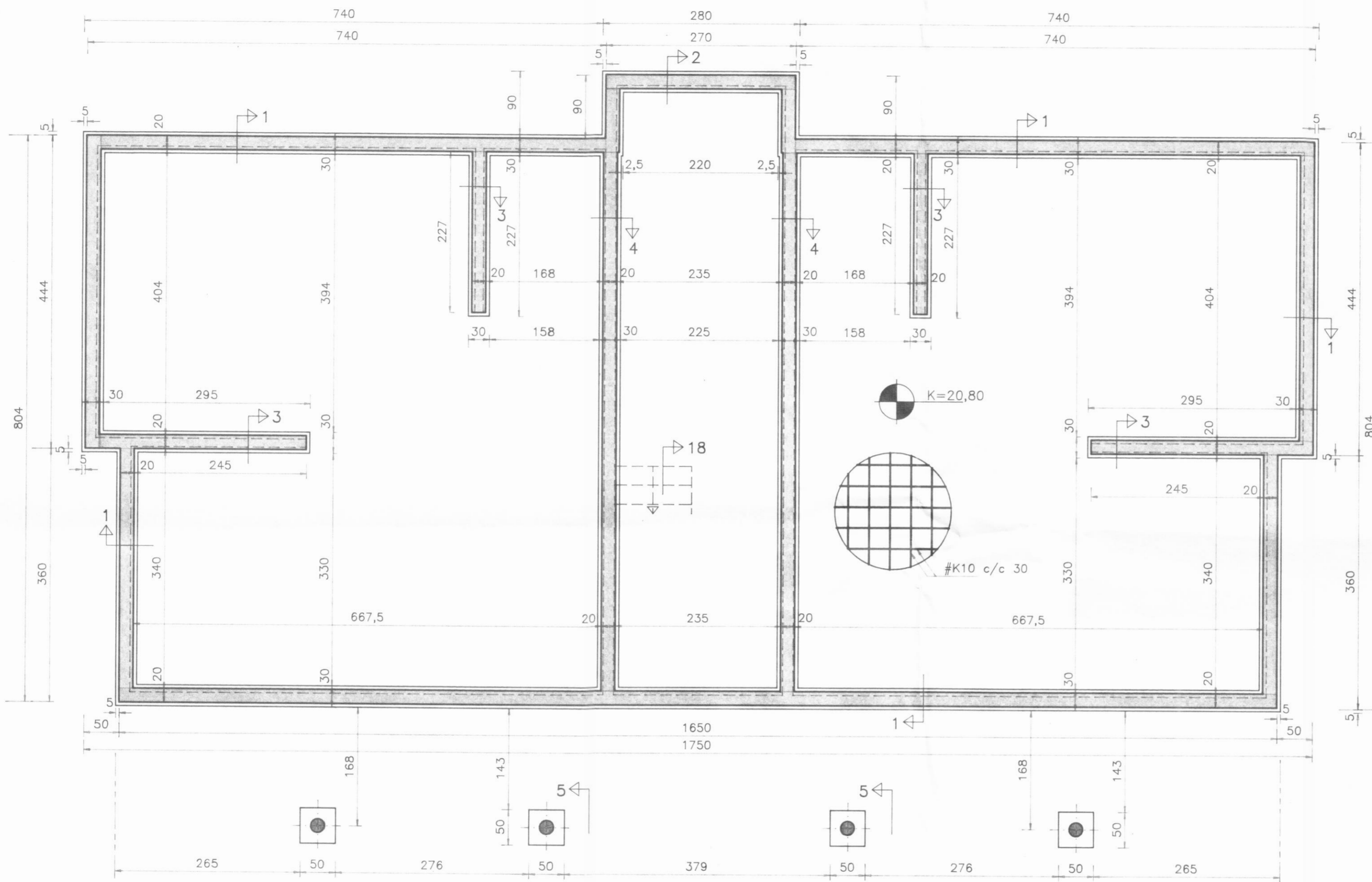
UNDIRSTÖÐUR GRUNNMYND mkv. 1:50
