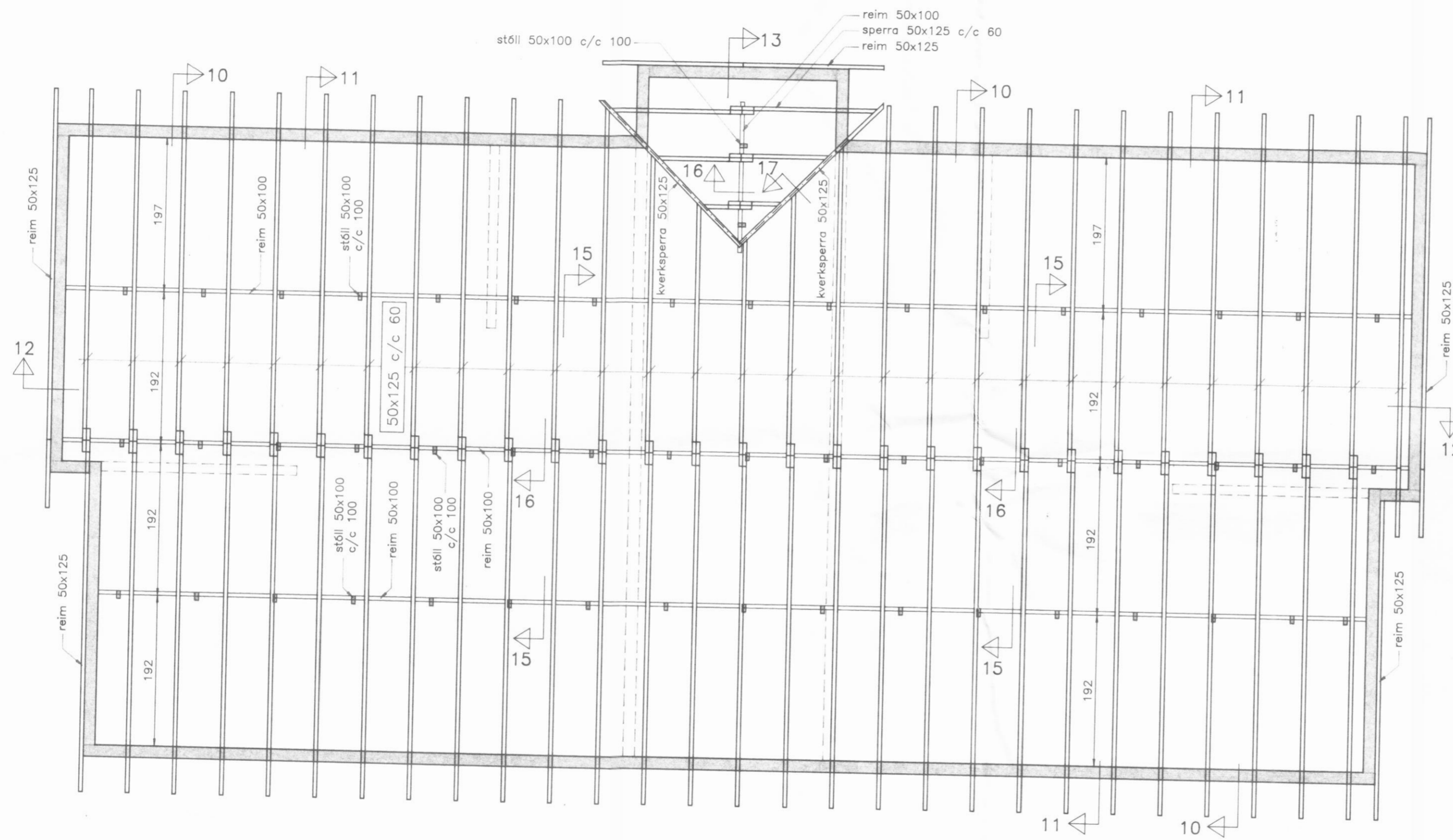
GRUNNMYND ÞAKVIÐA mkv. 1:50
