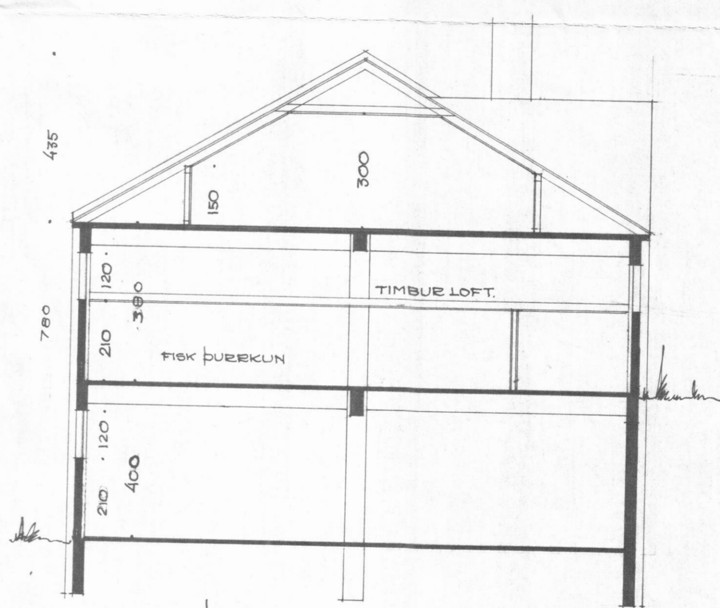
PYERSKURÐUR "B-B"
