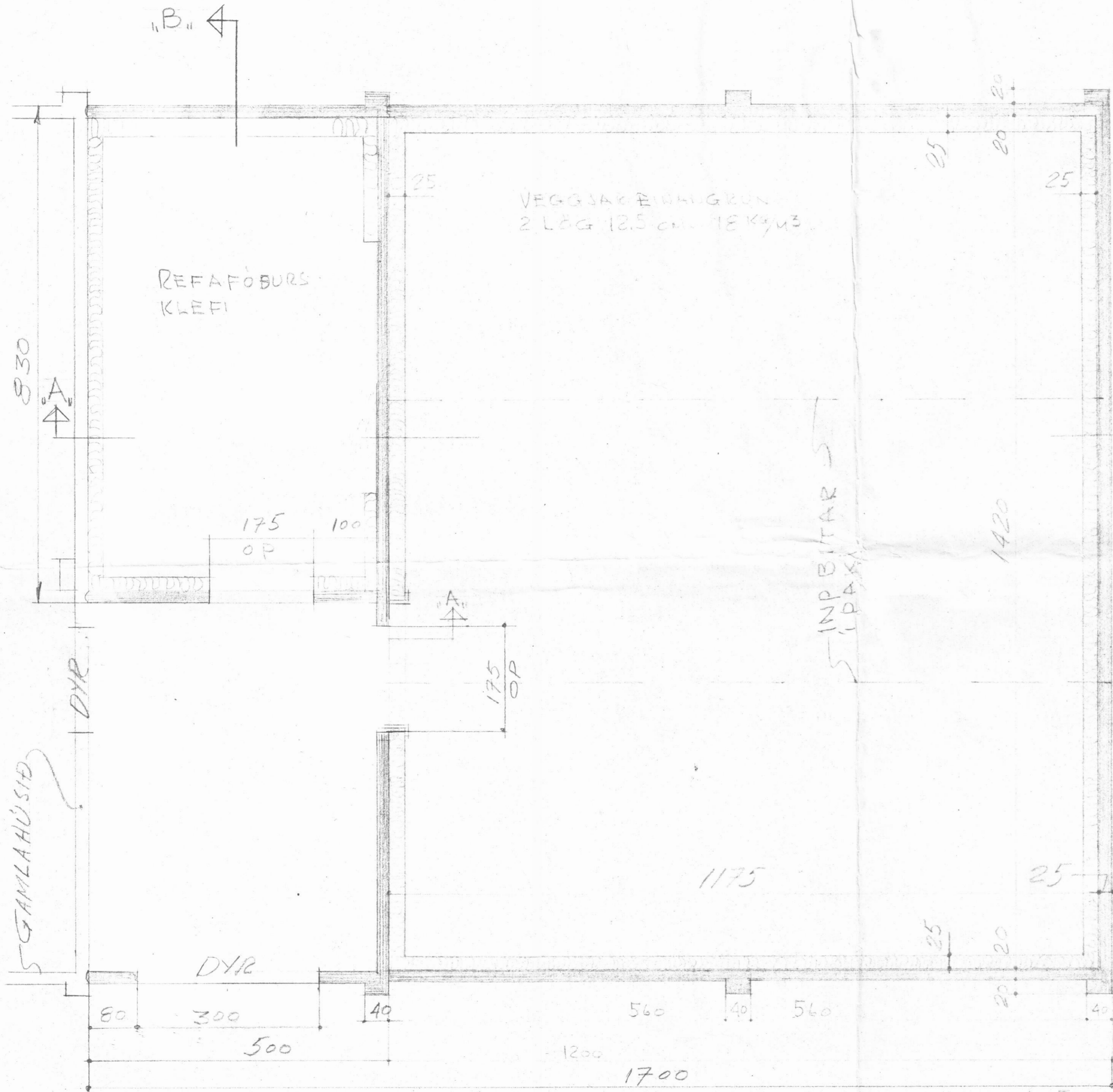
GRUNNMYND 1:50
