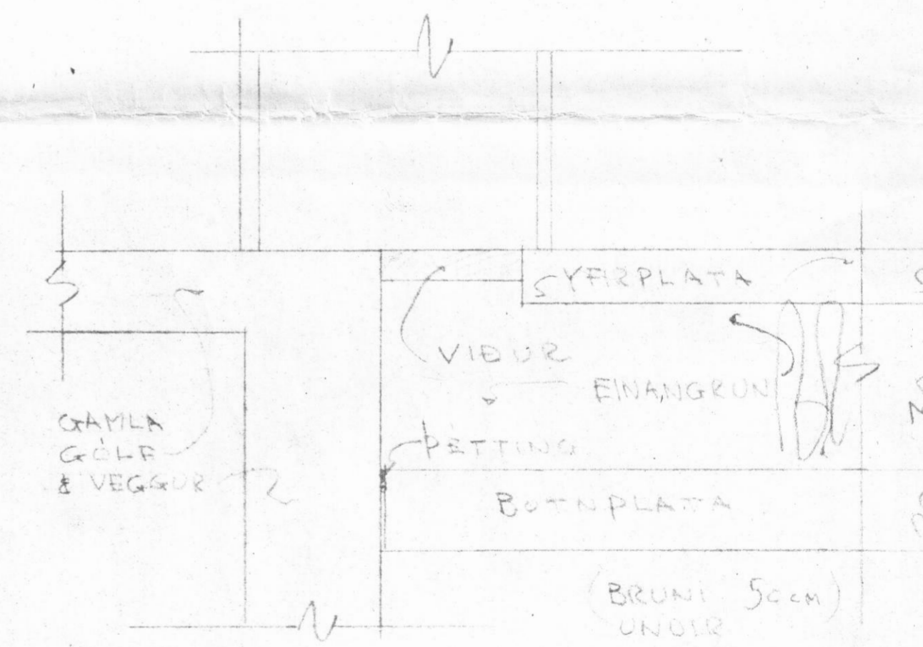
SKURÐUR „A“ 1:10
