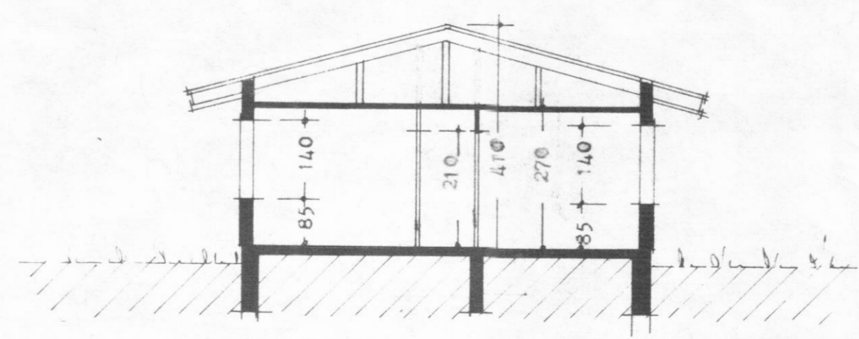
skurður B-B
