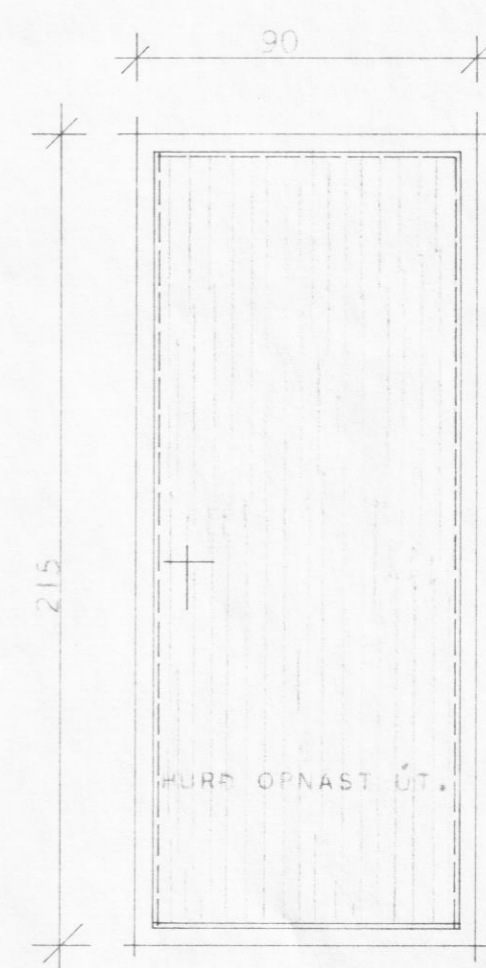
1 STK. ÞILGEYMSLURDUR.
