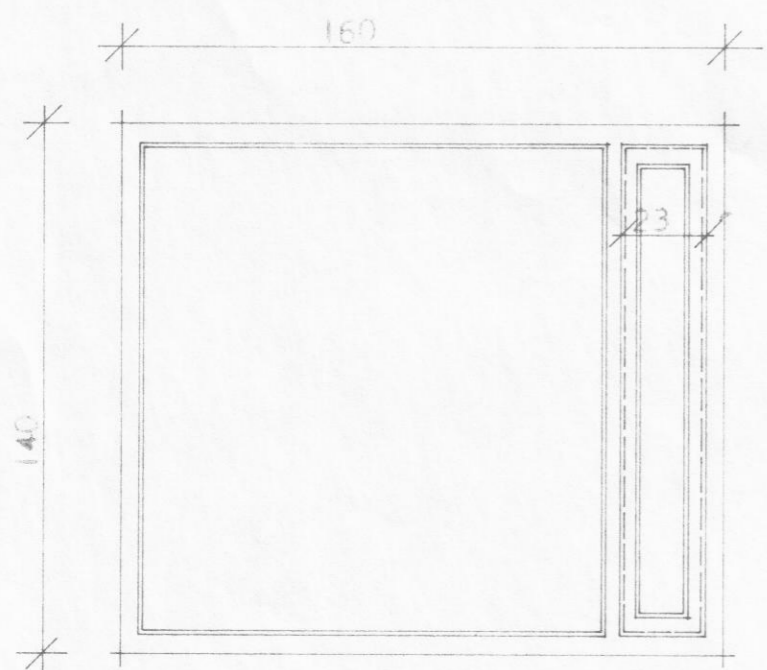
6 STK. HERBERGISLUGGAR.
