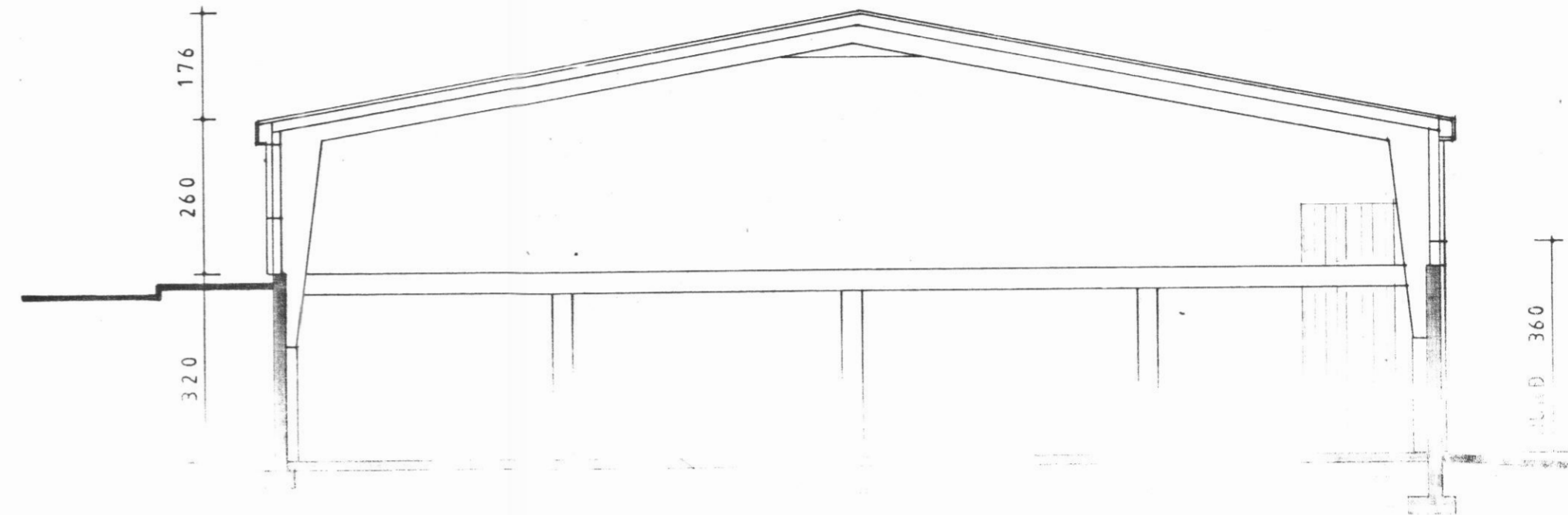
SNEIÐING B-B
