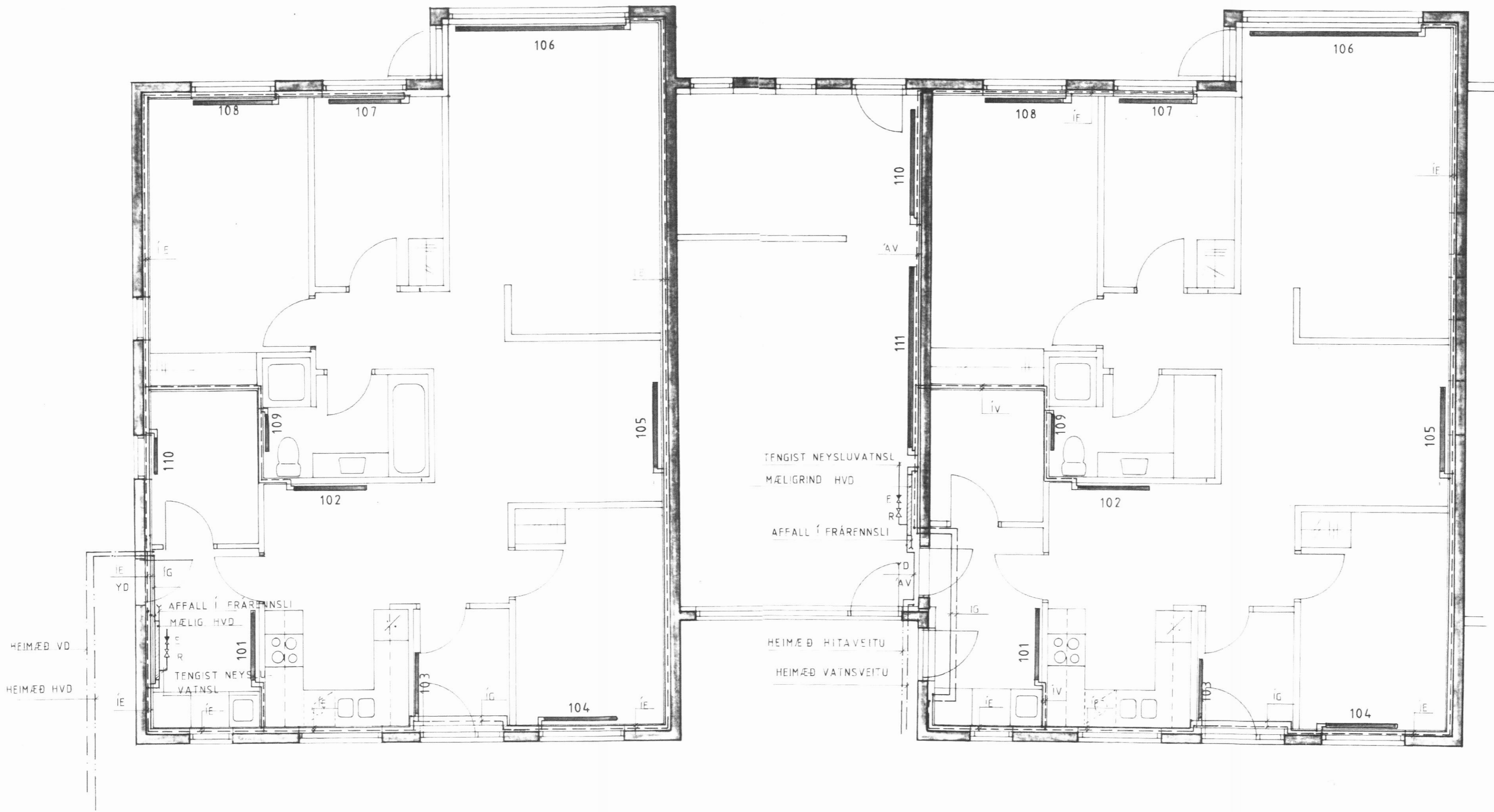
GRUNNMYND 1:50
