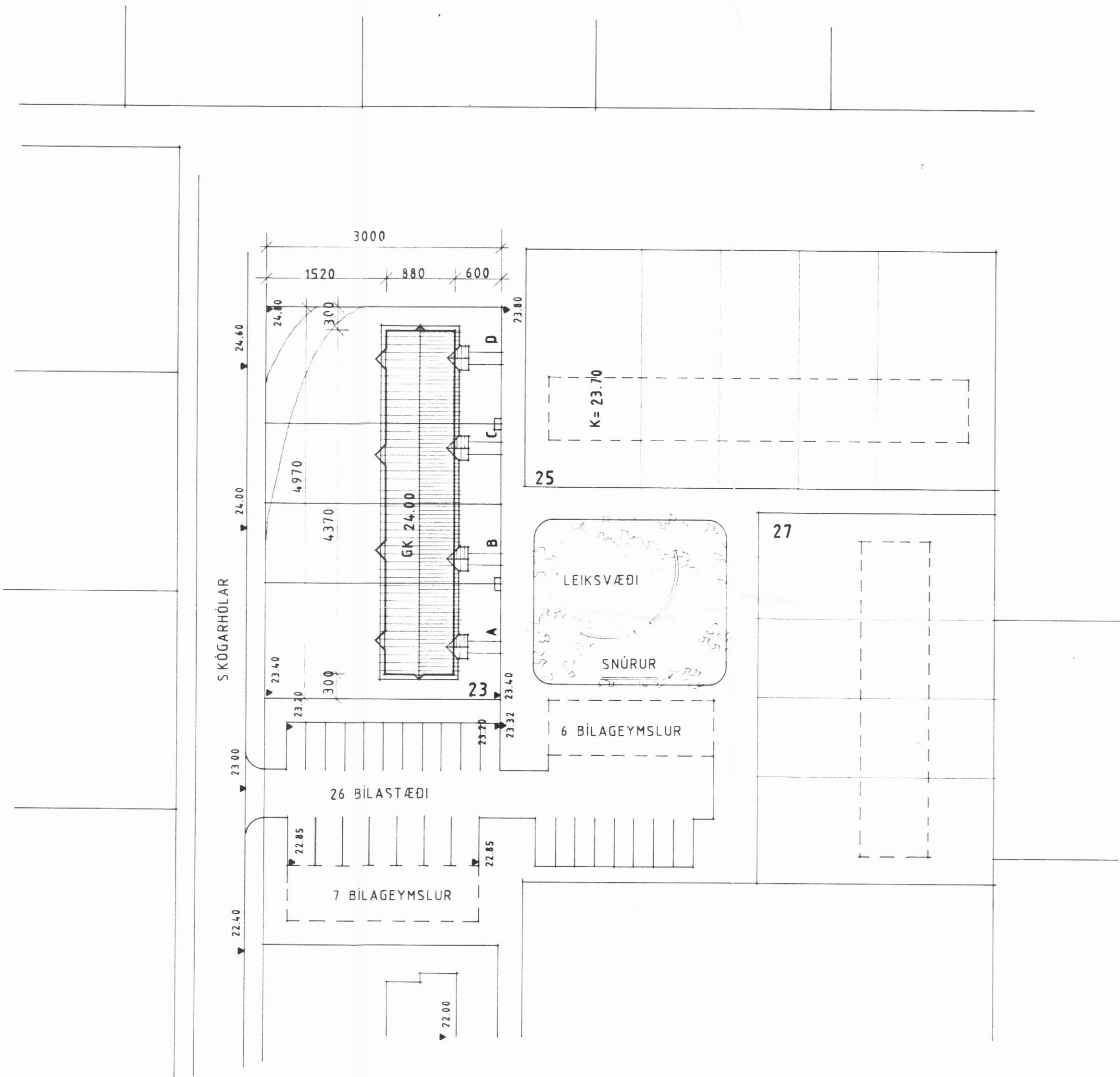
AFSTÖÐUMYND M 1:500
