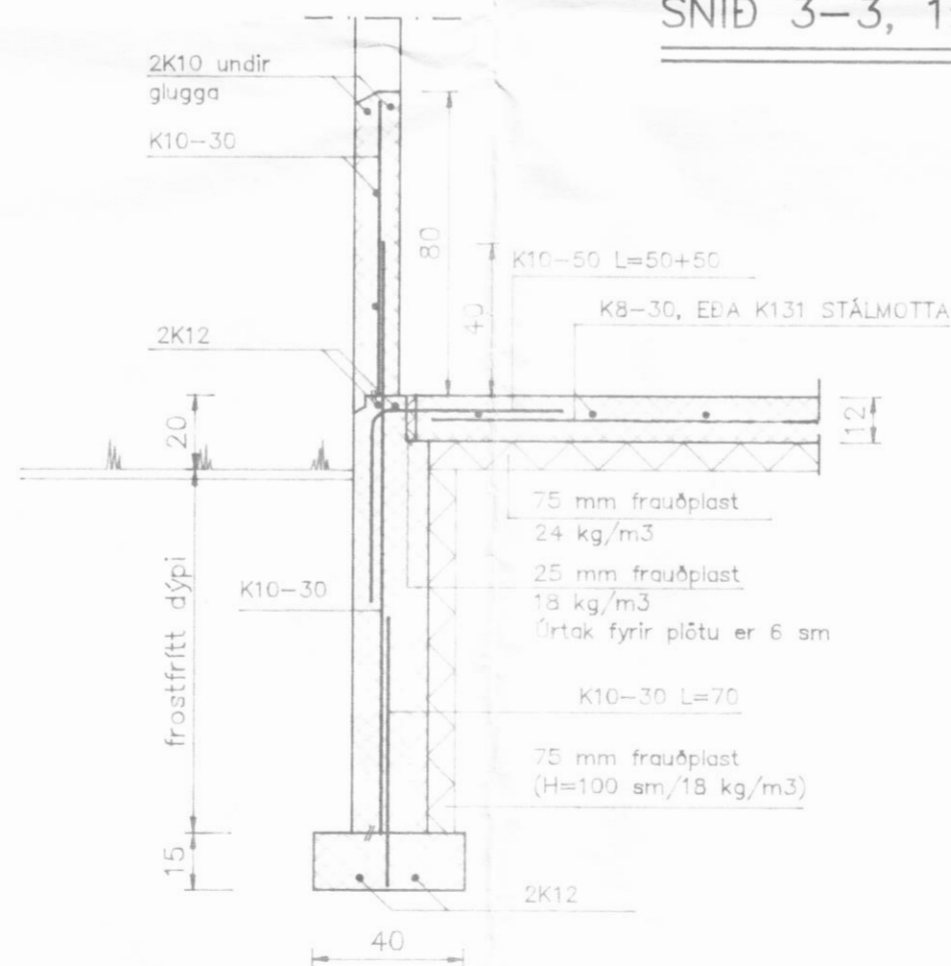
SNID 3-3, 1:20
