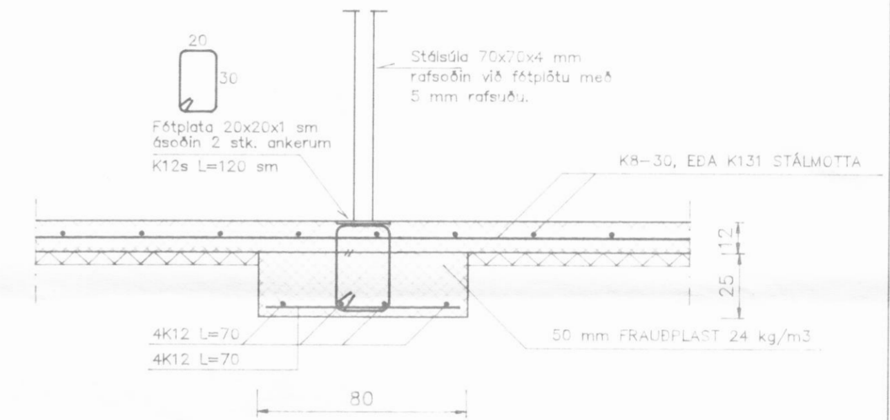
Undirstaða U1, 1:20
