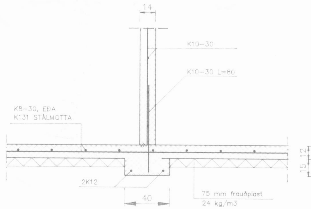
SNID 2-2, 1:20
