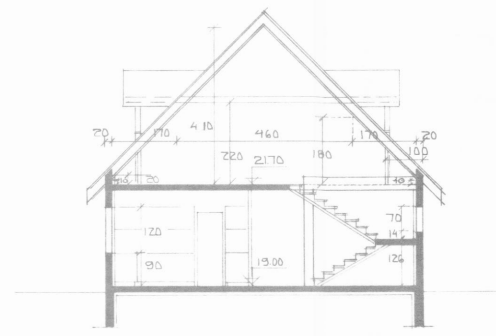
SNID A-A 1:100
