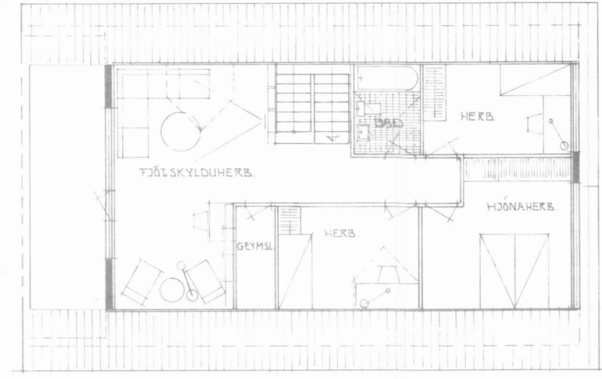
GRUNNMYND RISHEÐAR 1:100
