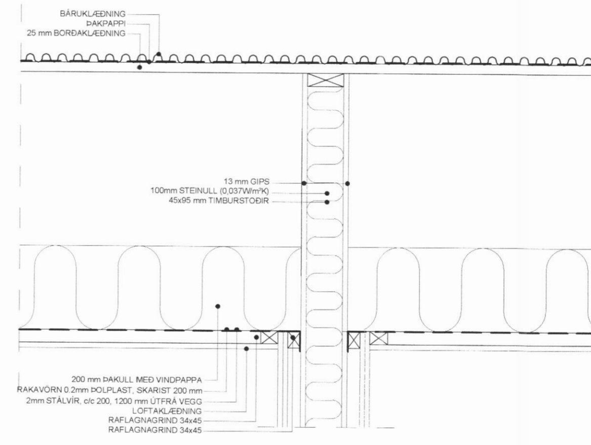
D2 LÓÐRÉTT SNIÐ - EI60 VEGGUR 1:10
