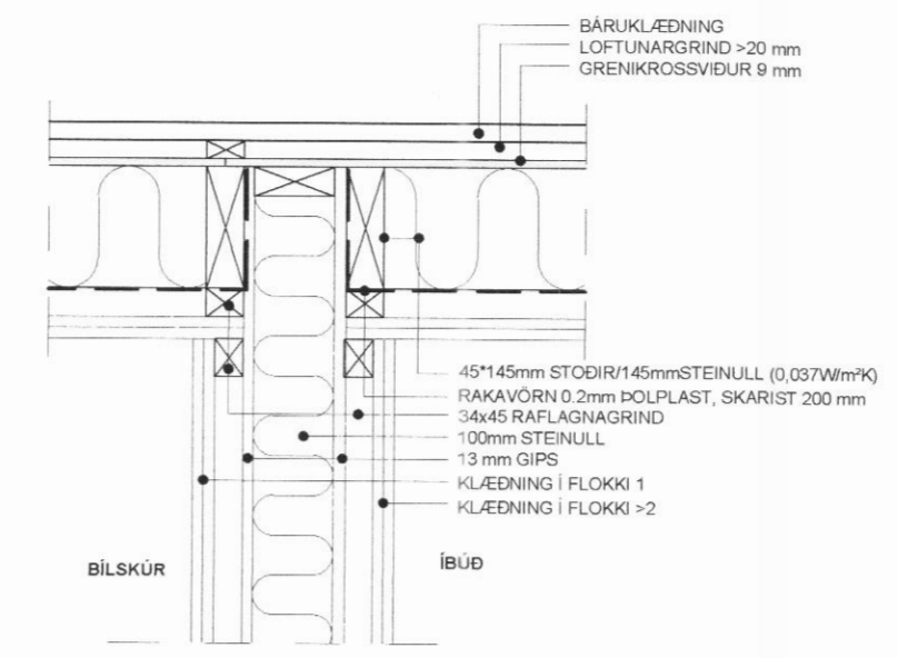
D4 DEILI - EI60 / 44 DB VEGGUR AÐ ÚTVEGG 1:10
