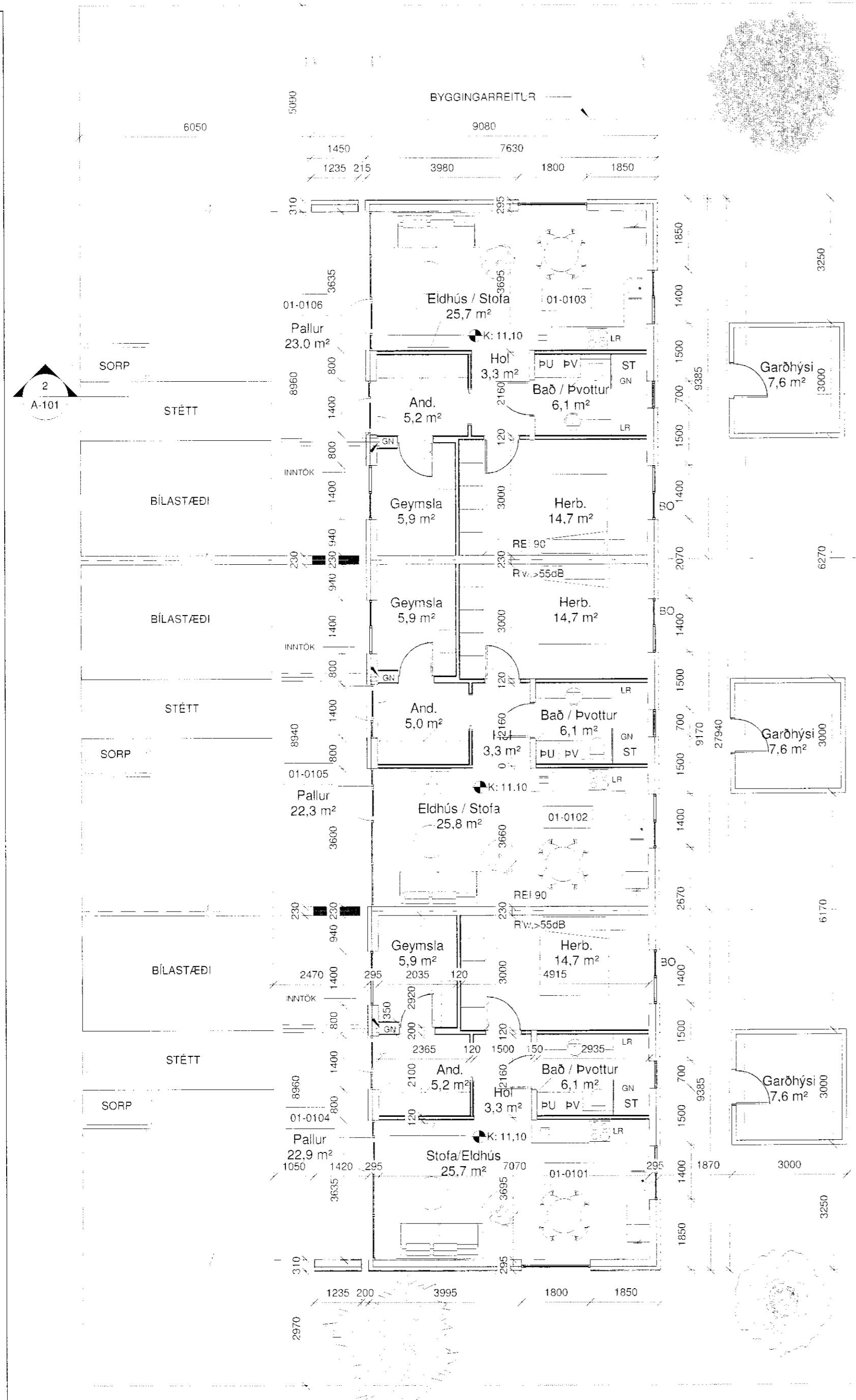
1 Grunnmynd 1 : 100
