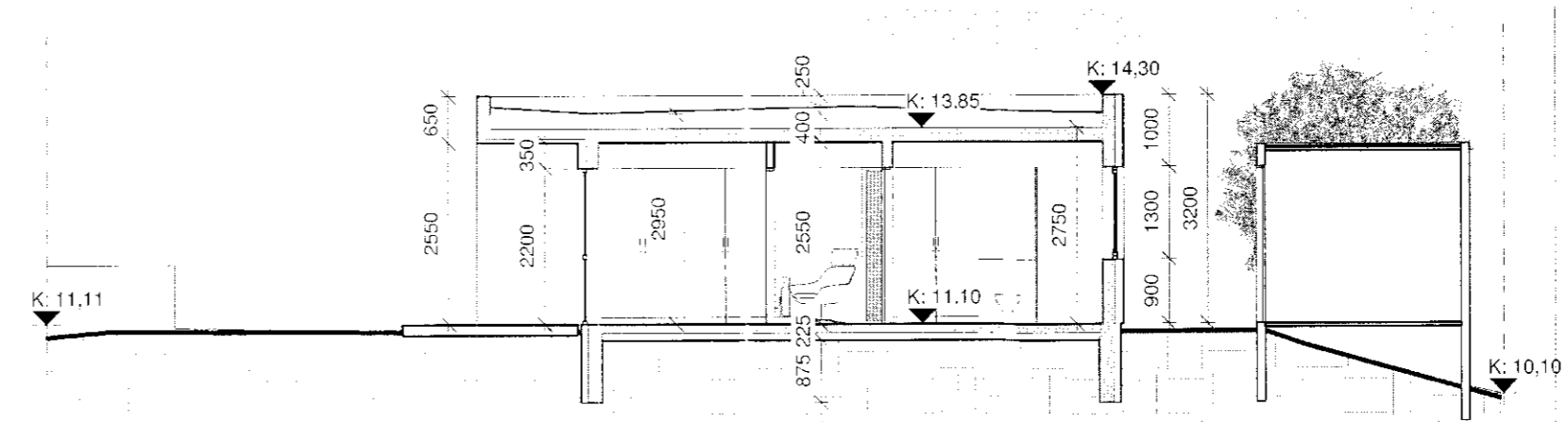
2 Snið A-A 1 : 100
