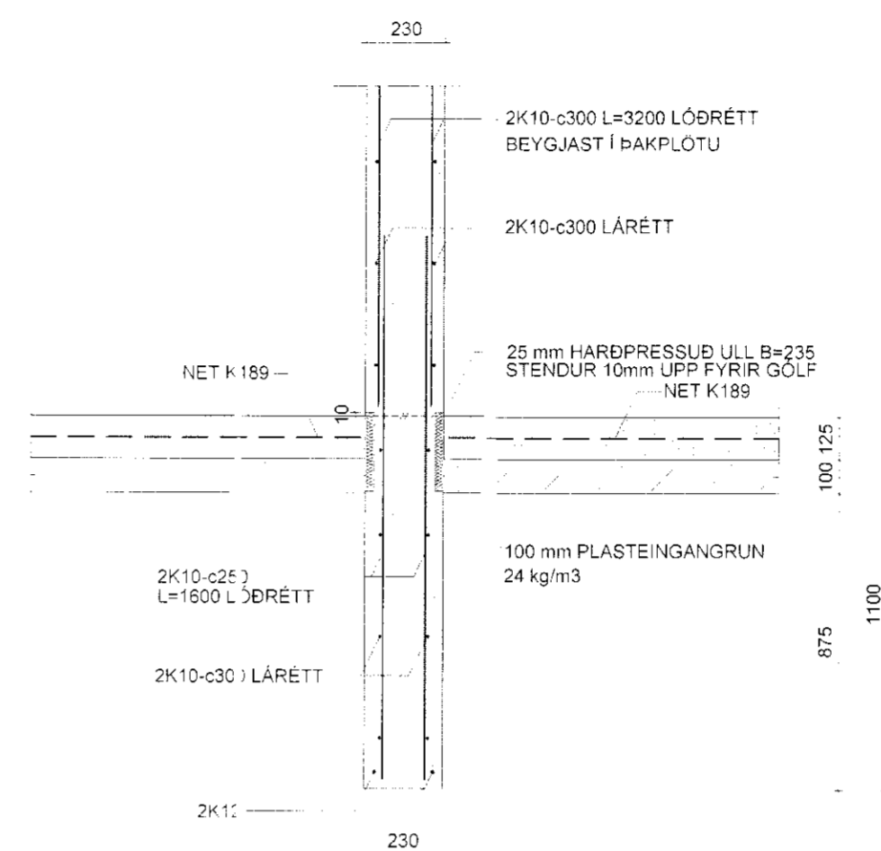
3 Snið 1:20
