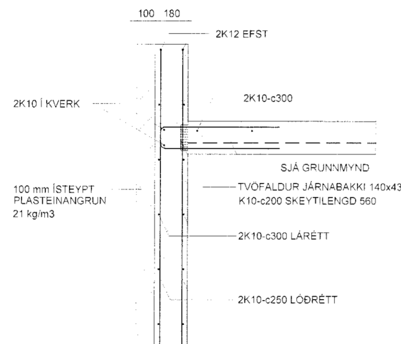
10 Snið 1:20
