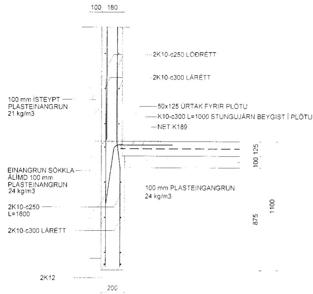
1 Snið 1:20
