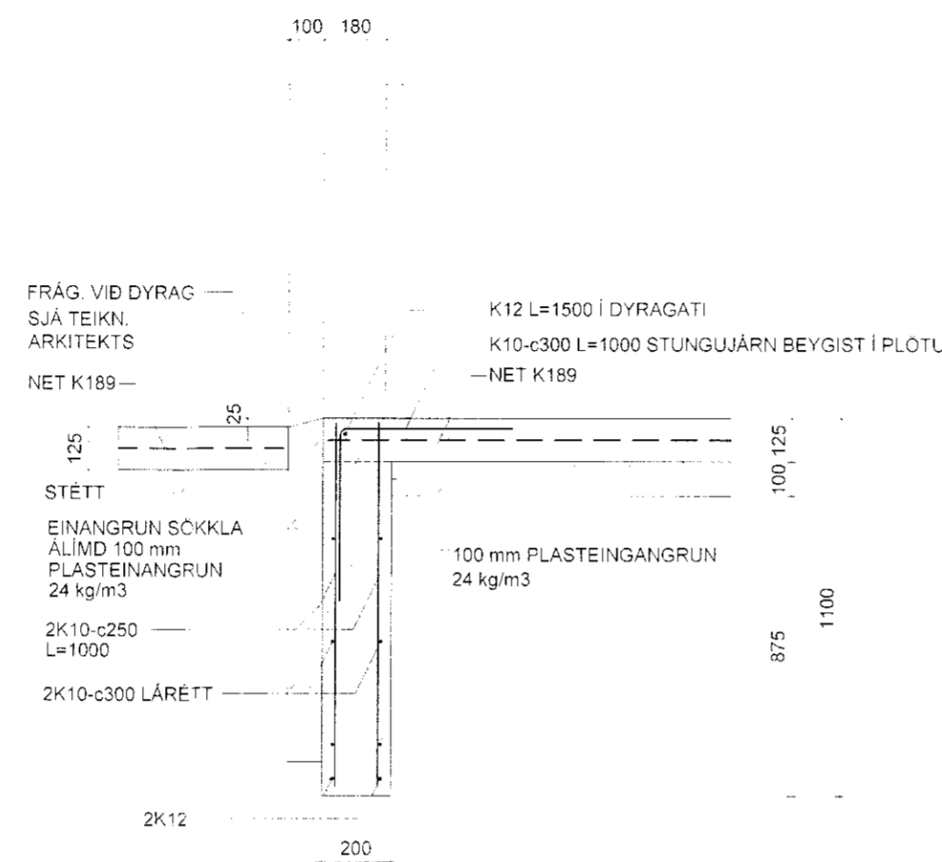
2 Snið 1:20
