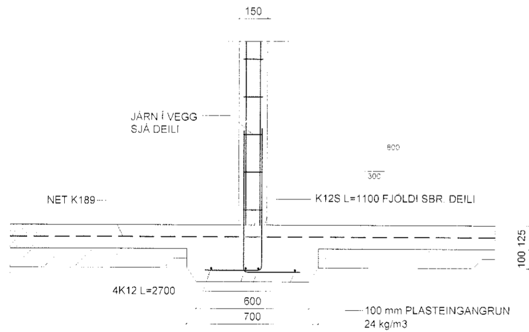
4 Snið 1:20
