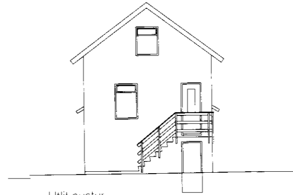
Útlit austur 1:100
