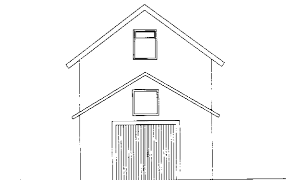
Útlit vestur 1:100
