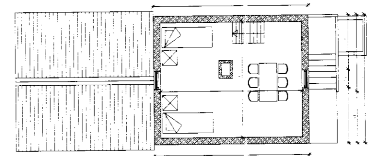
Grunnmynd 2. hæð 1:100
