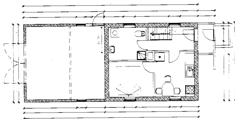
Grunnmynd kjallari 1:100
