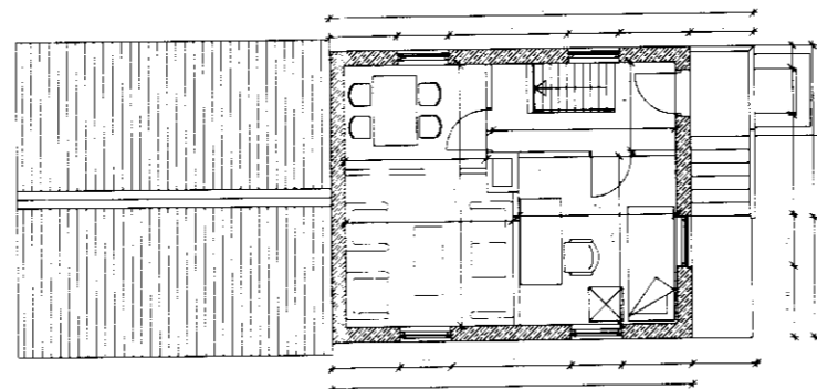
Grunnmynd 1. hæð 1:100
