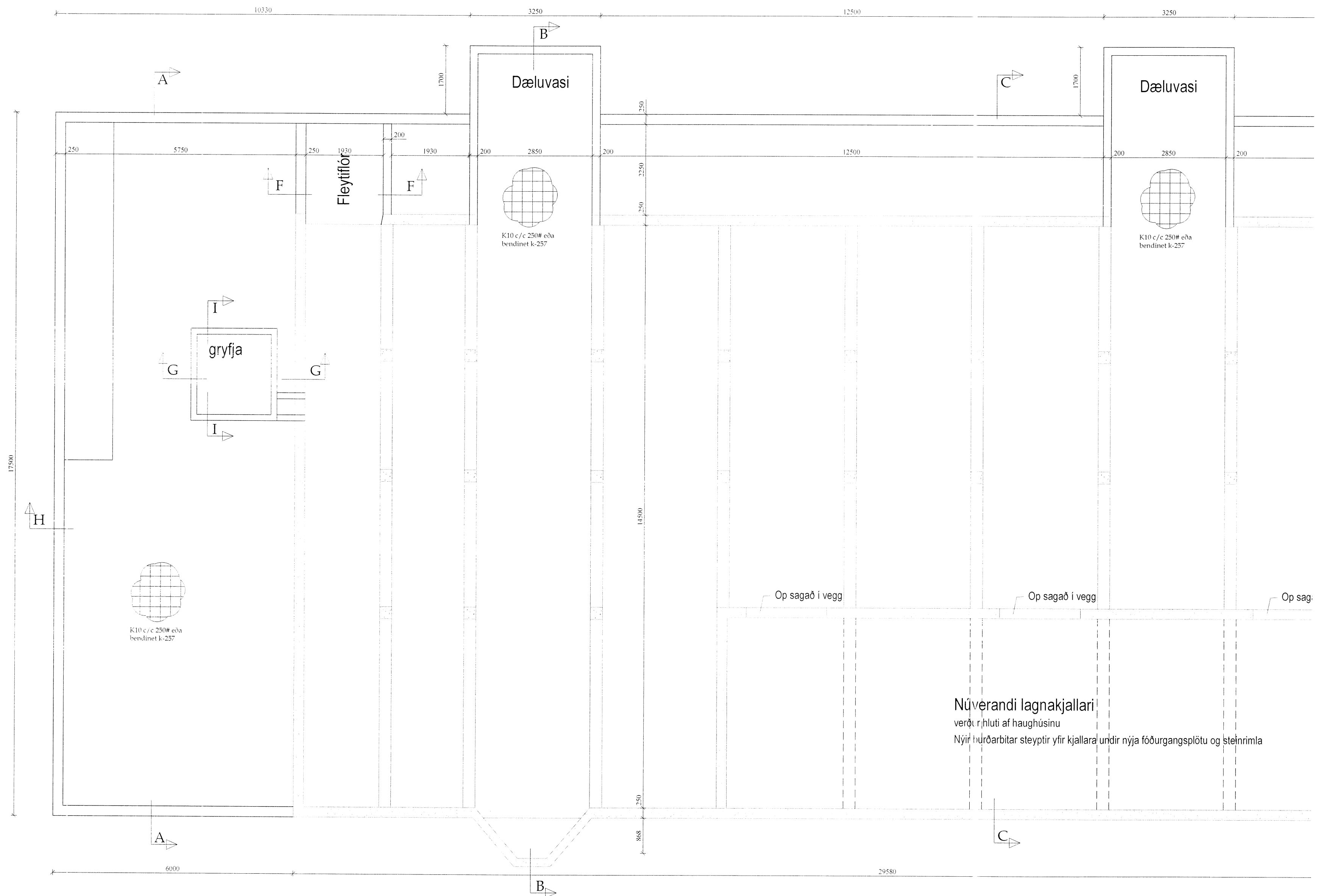
Burðarvirki-Grunnmynd, mk. 1:50
