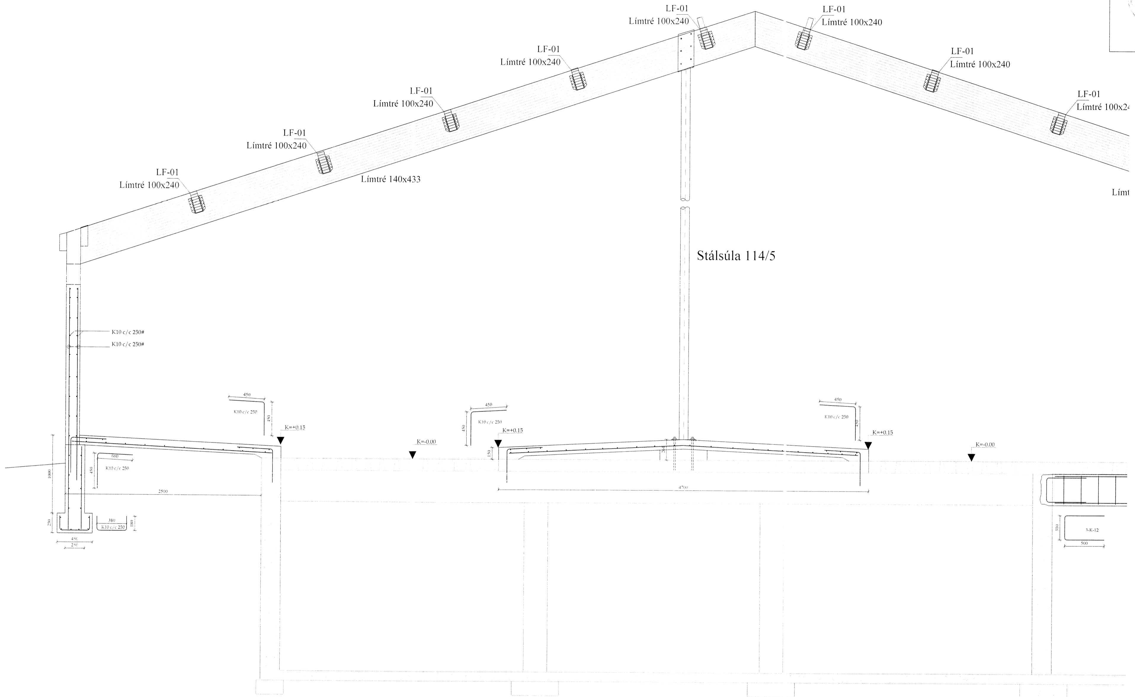
Þversnið C-C mk. 1:20
