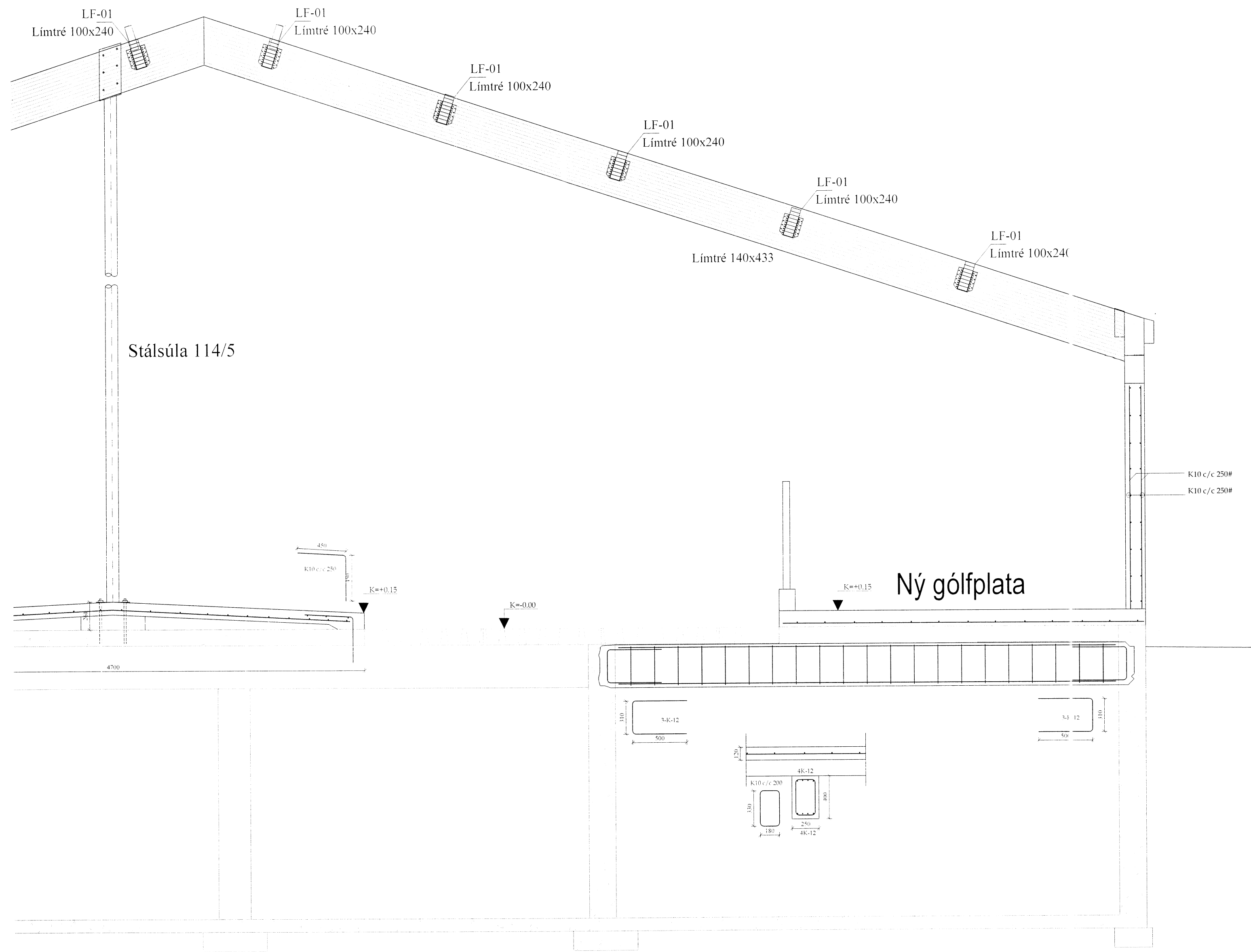
Þversnið C-C hluti 2 mk. 1:20
