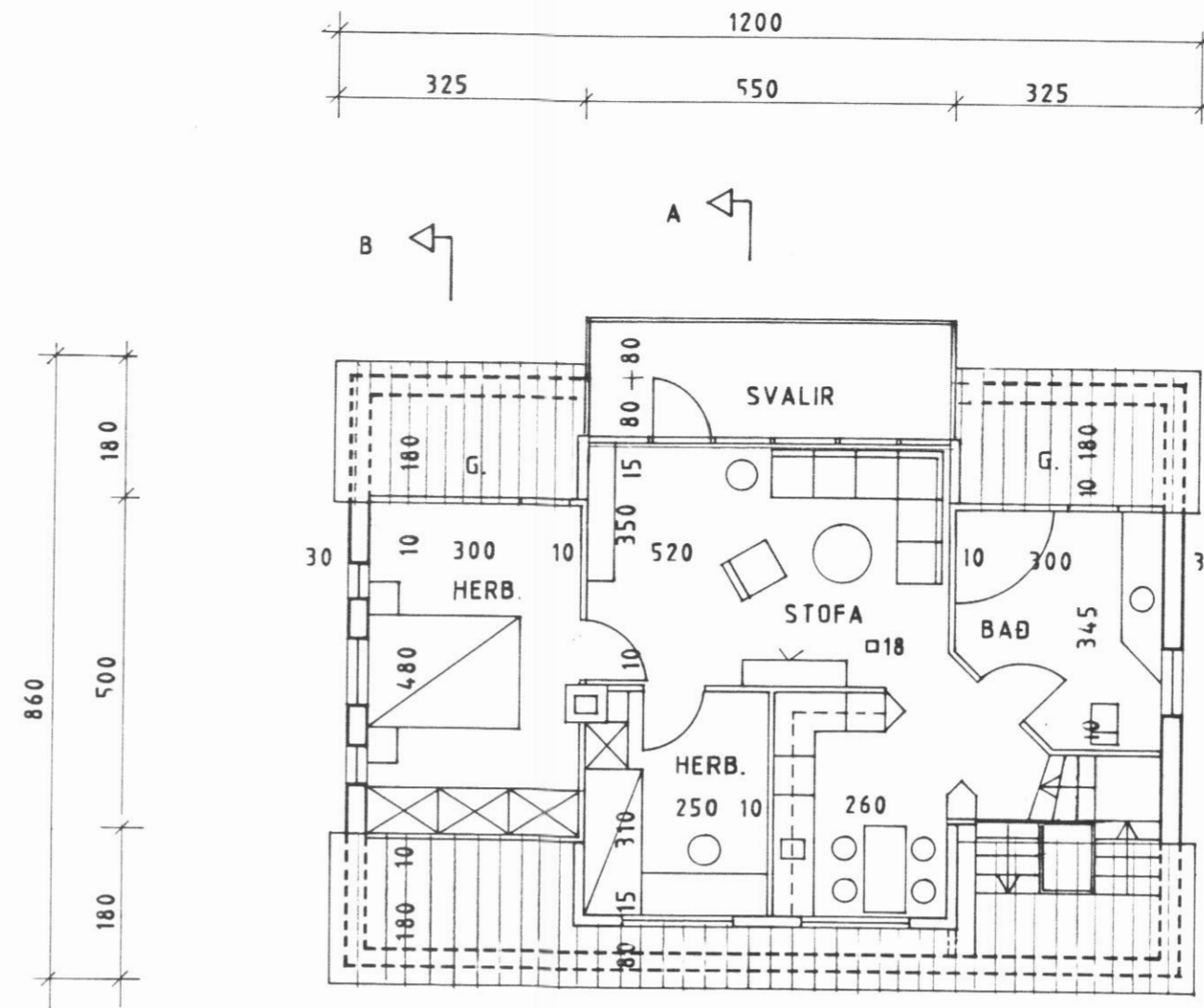
GRUNNMYND RISHÆÐAR
