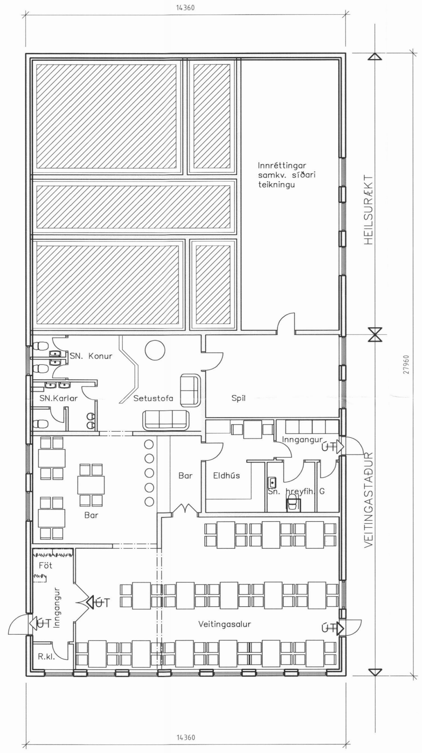
GRUNNMYND KJALLARA--INNRETTINGAR
