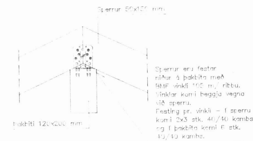
Sérm. 3, 1:10
