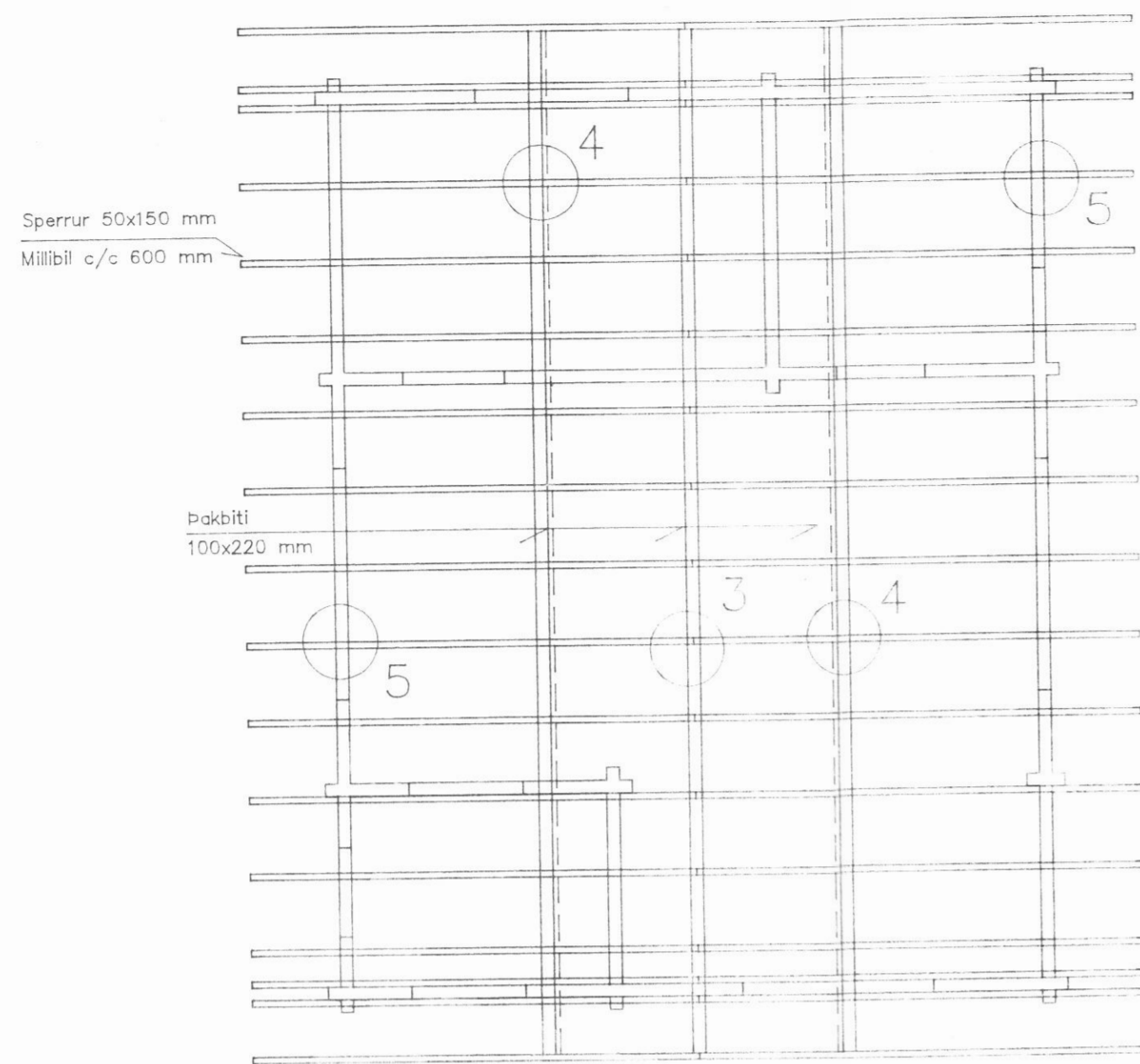
Grunnm. þakbita.
