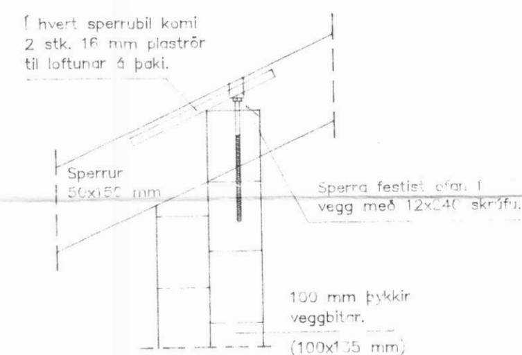
Sérm. 3, 1:10
