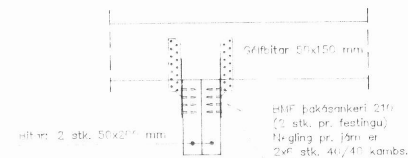
Sérm. 2, 1:10
