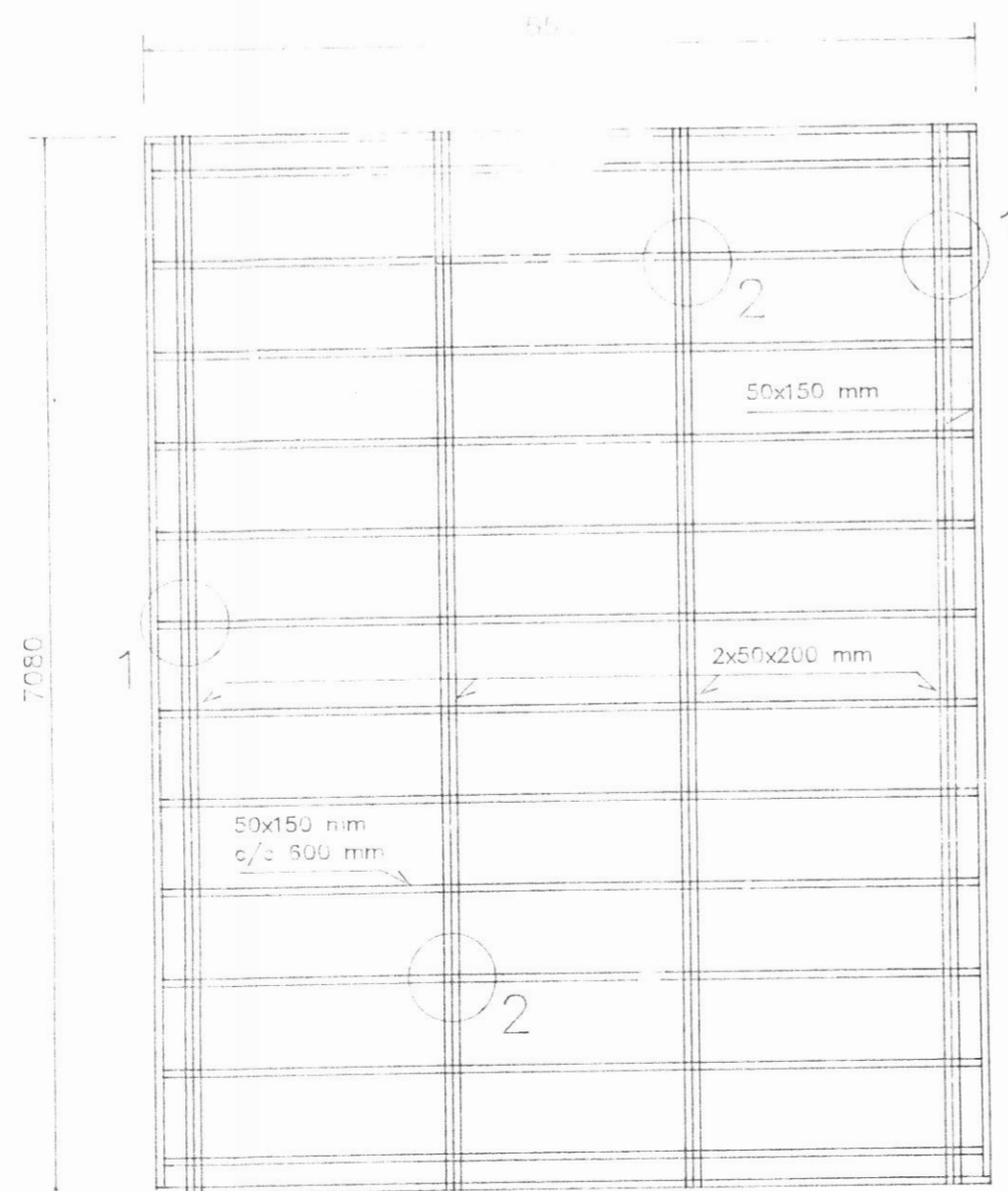
Grunnm. gólfbita.
