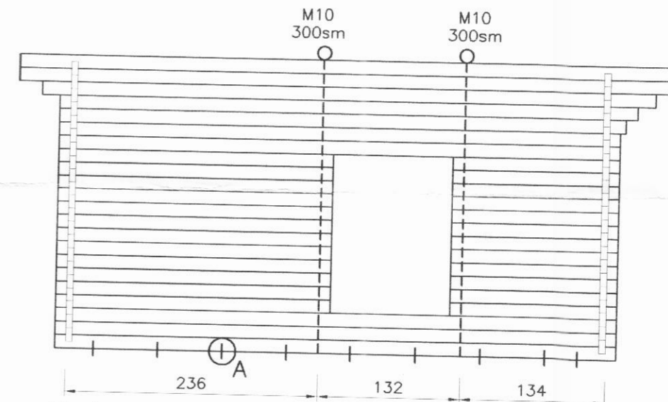
Vesturhlið. Mkv. 1:50
