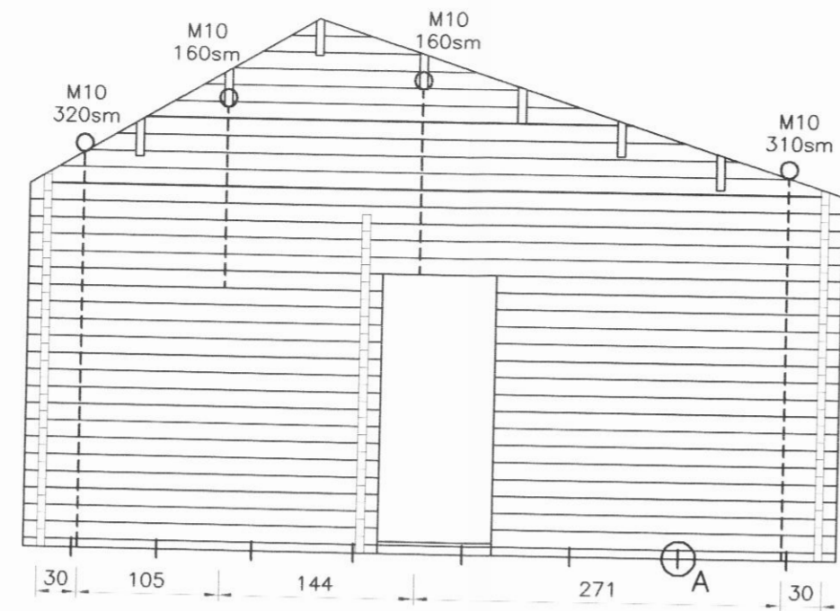
Norðurhlið. Mkv. 1:50
