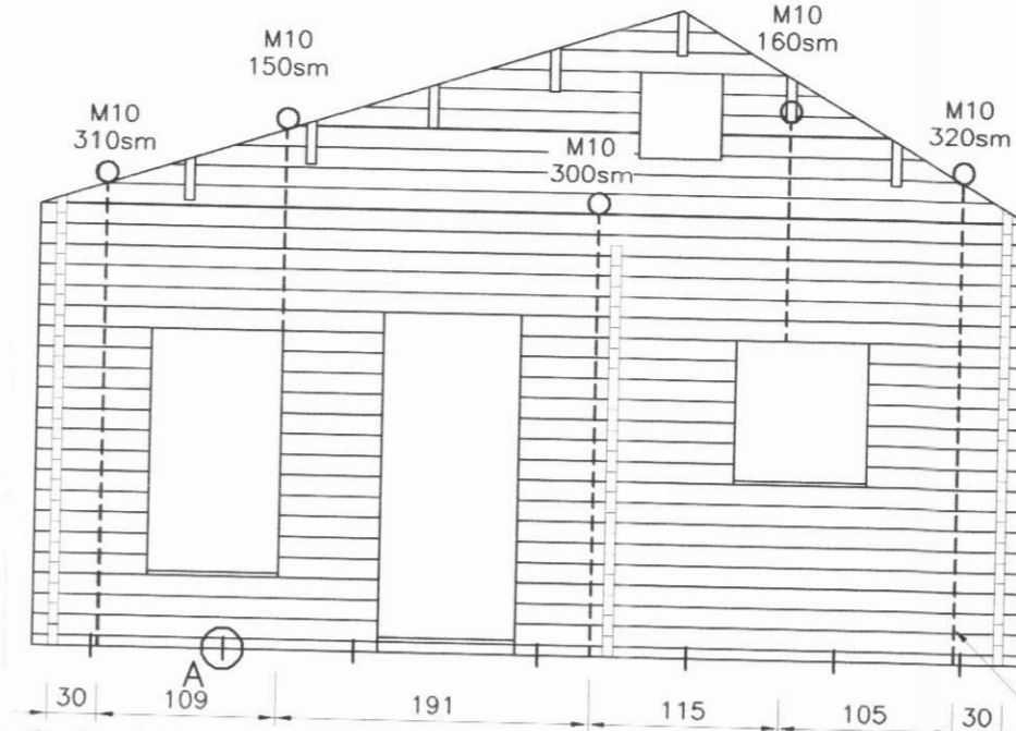
Suðurhlið. Mkv. 1:50
