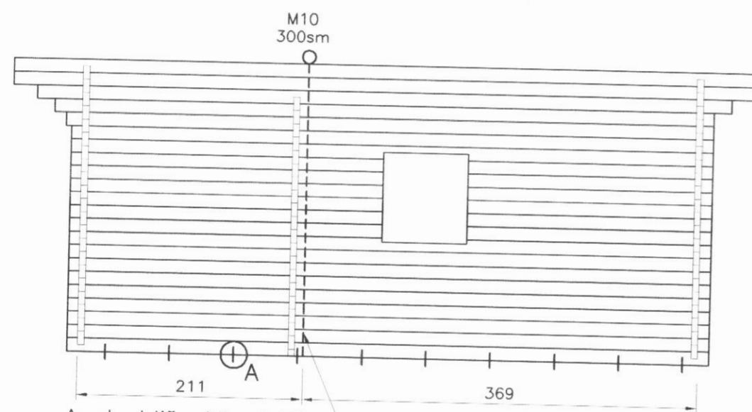
Austurhlið. Mkv. 1:50
