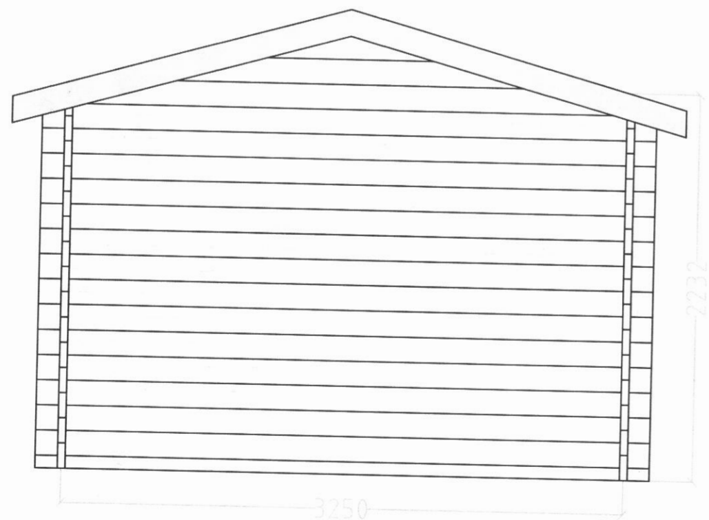
Snið C-C
