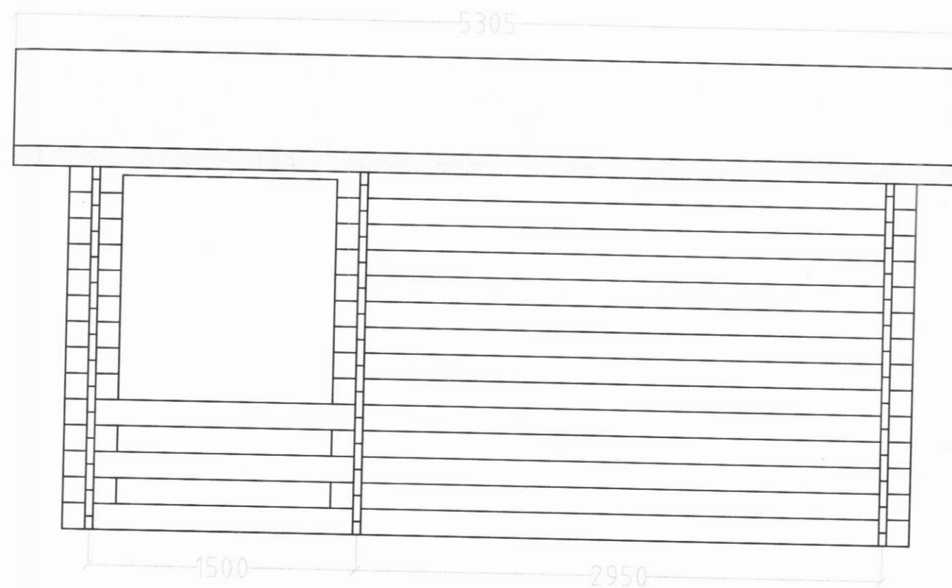
Snið D-D
