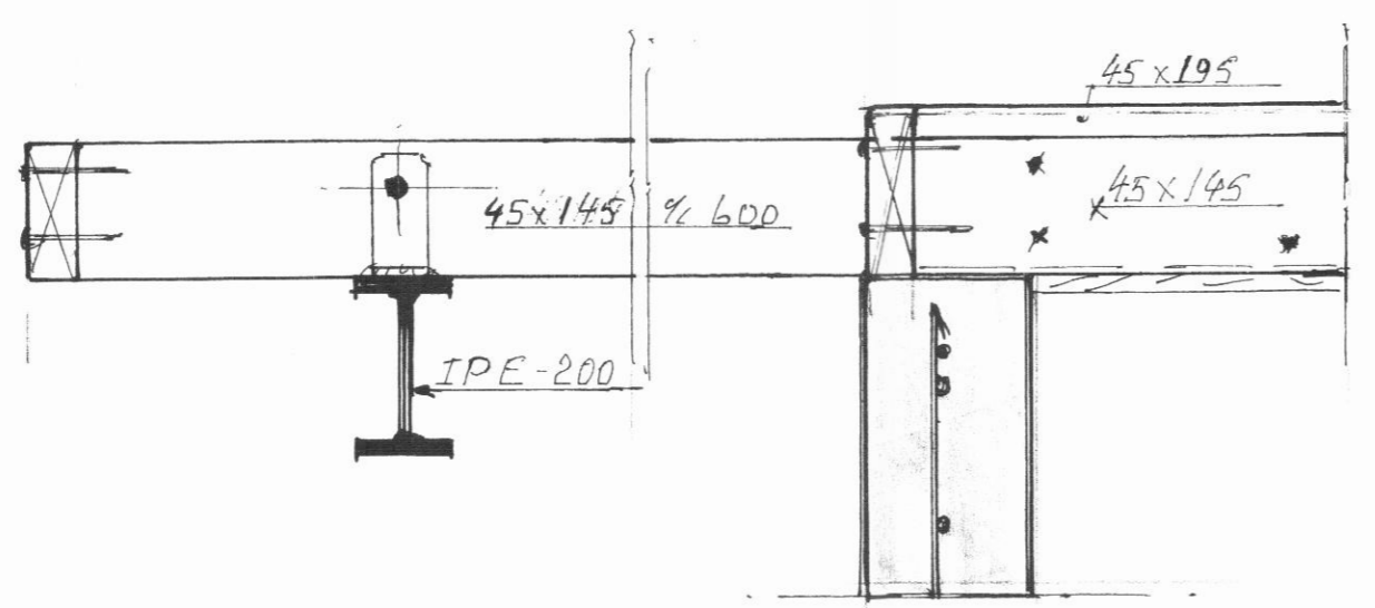
Frágangur gölfbita við innskot o.fl. Snid E-E; M1:10
