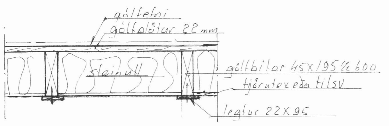
Frágangur gólfa; M1:10
