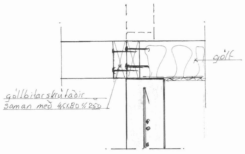
Samsetning tengibyggingar snid D-D; M1:10
