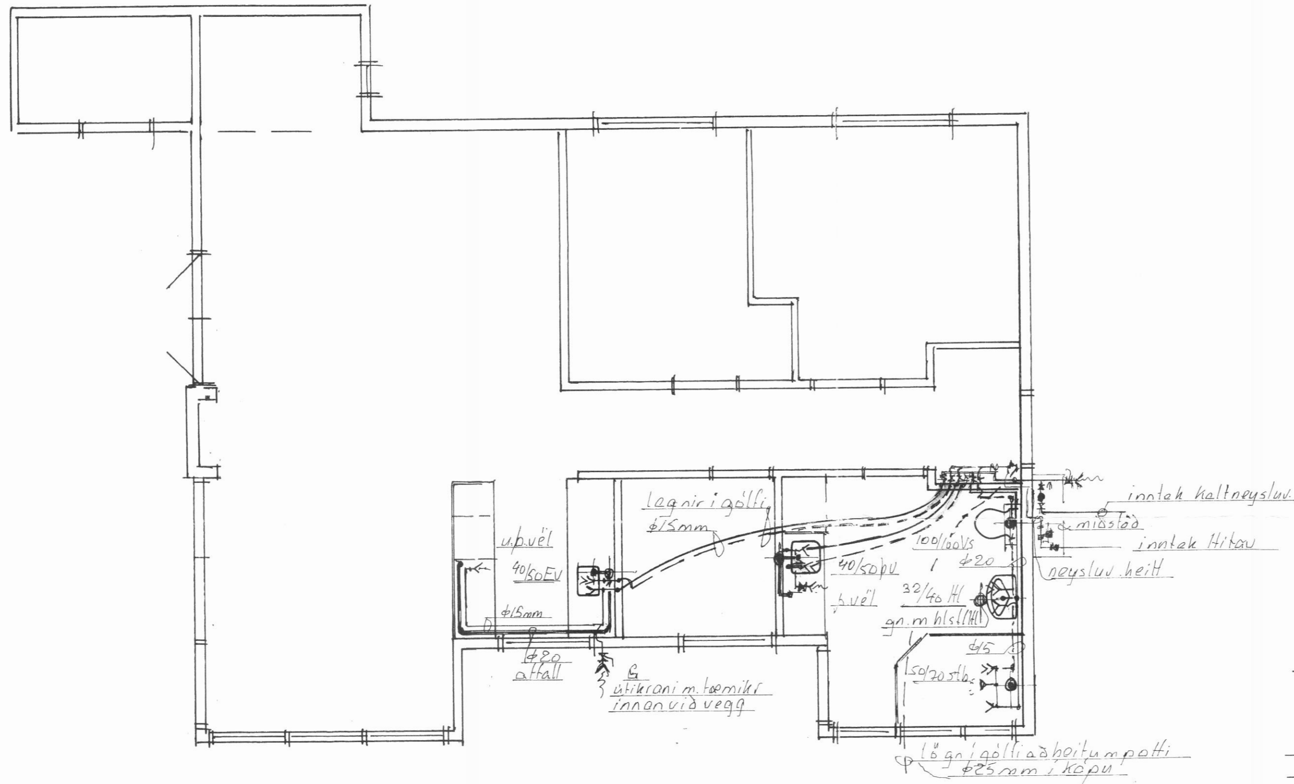
Neysluvatnslagnir; Grunnmynd; M 1:50
