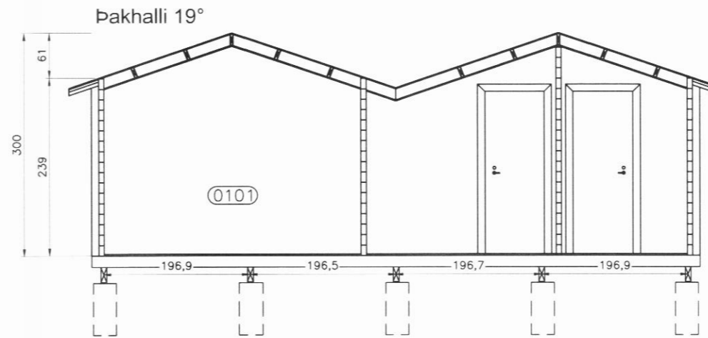
SNID A-A 1:50
