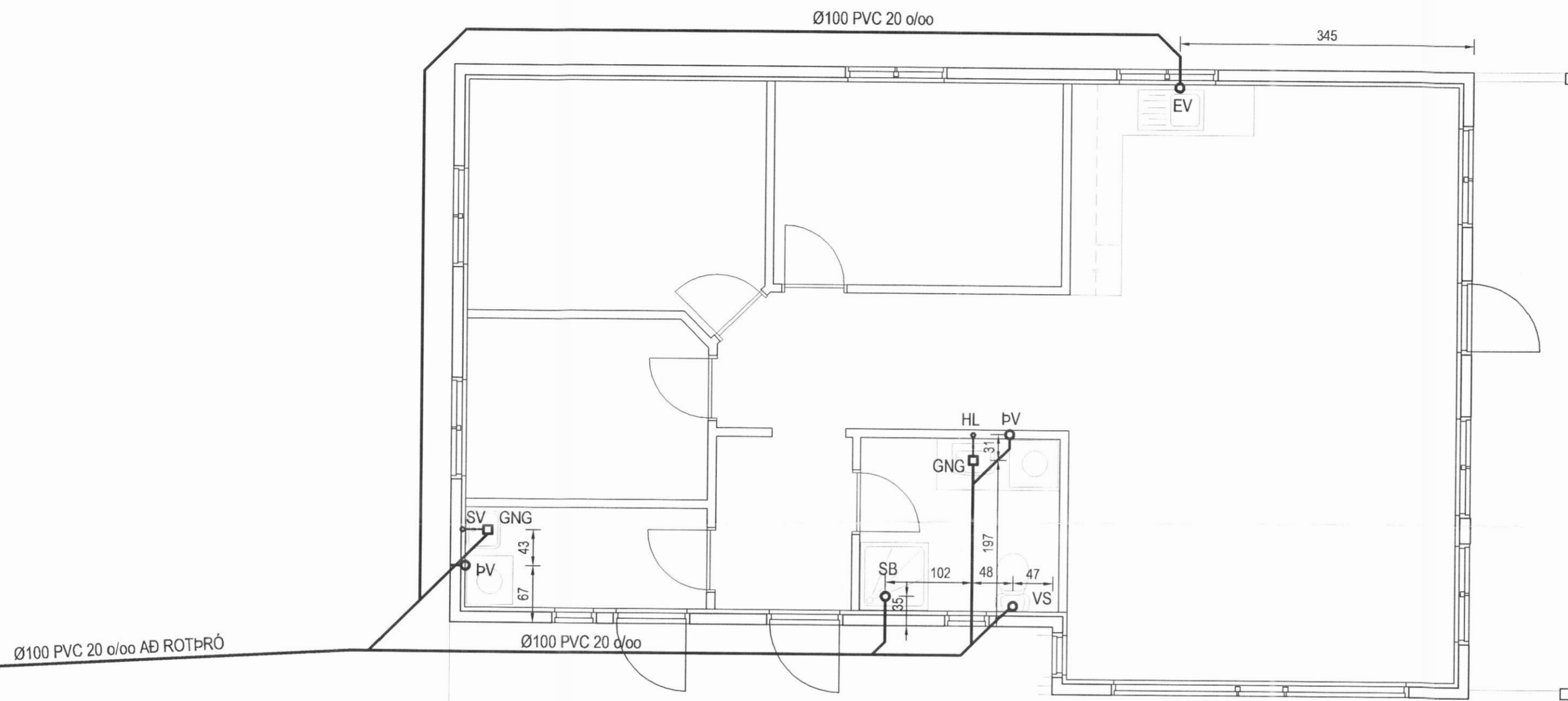
FRÁRENNSLISLAGNIR GRUNNMYND MKV. 1:50
