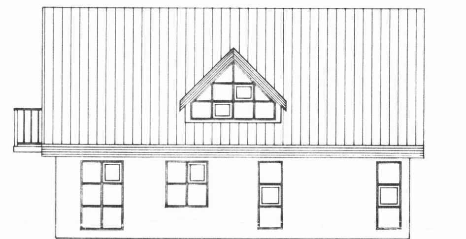
ÚTLITSMYND AUSTUR
