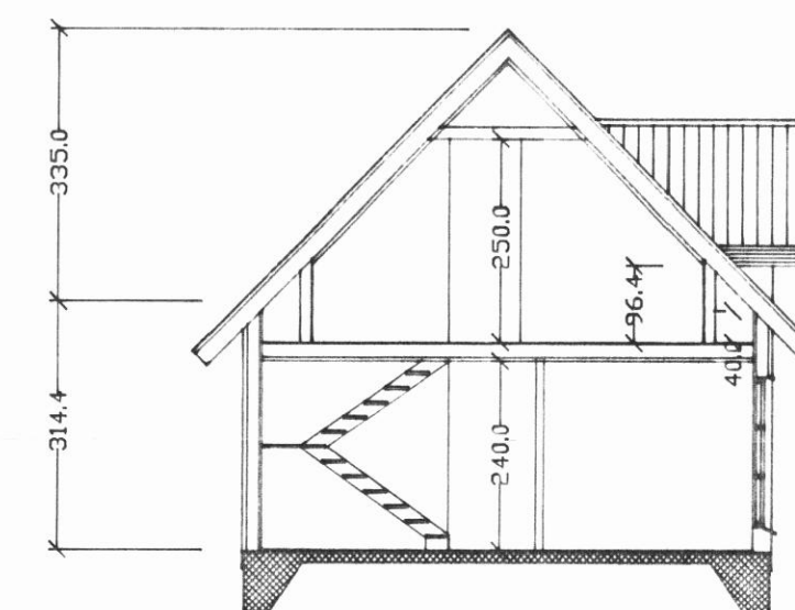
SNEIÐING A - A.
