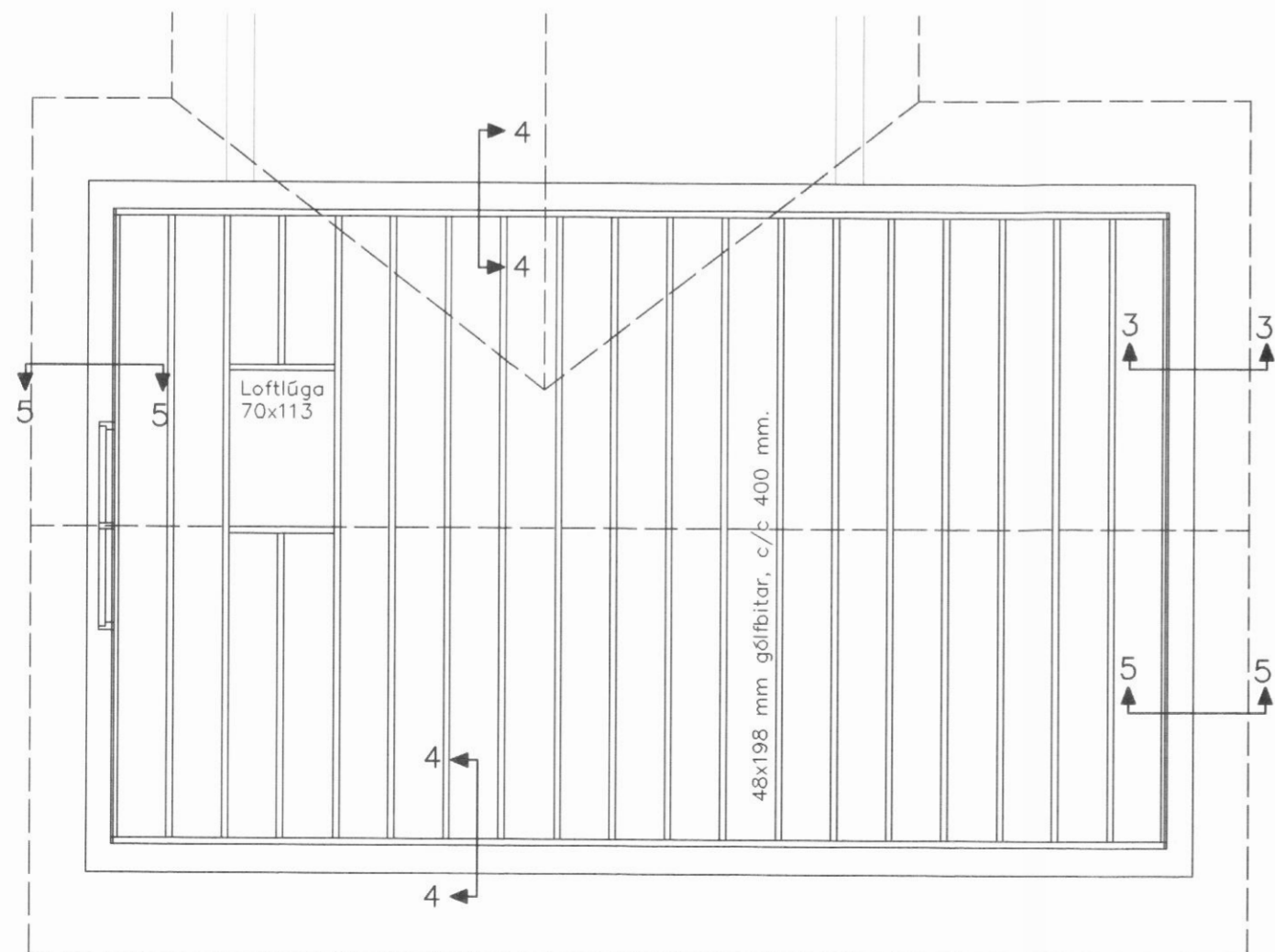
GÓLFBITAPLAN 1:50
