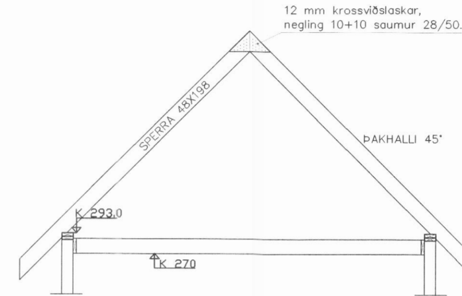
ÞAKSPERRA 1:50
