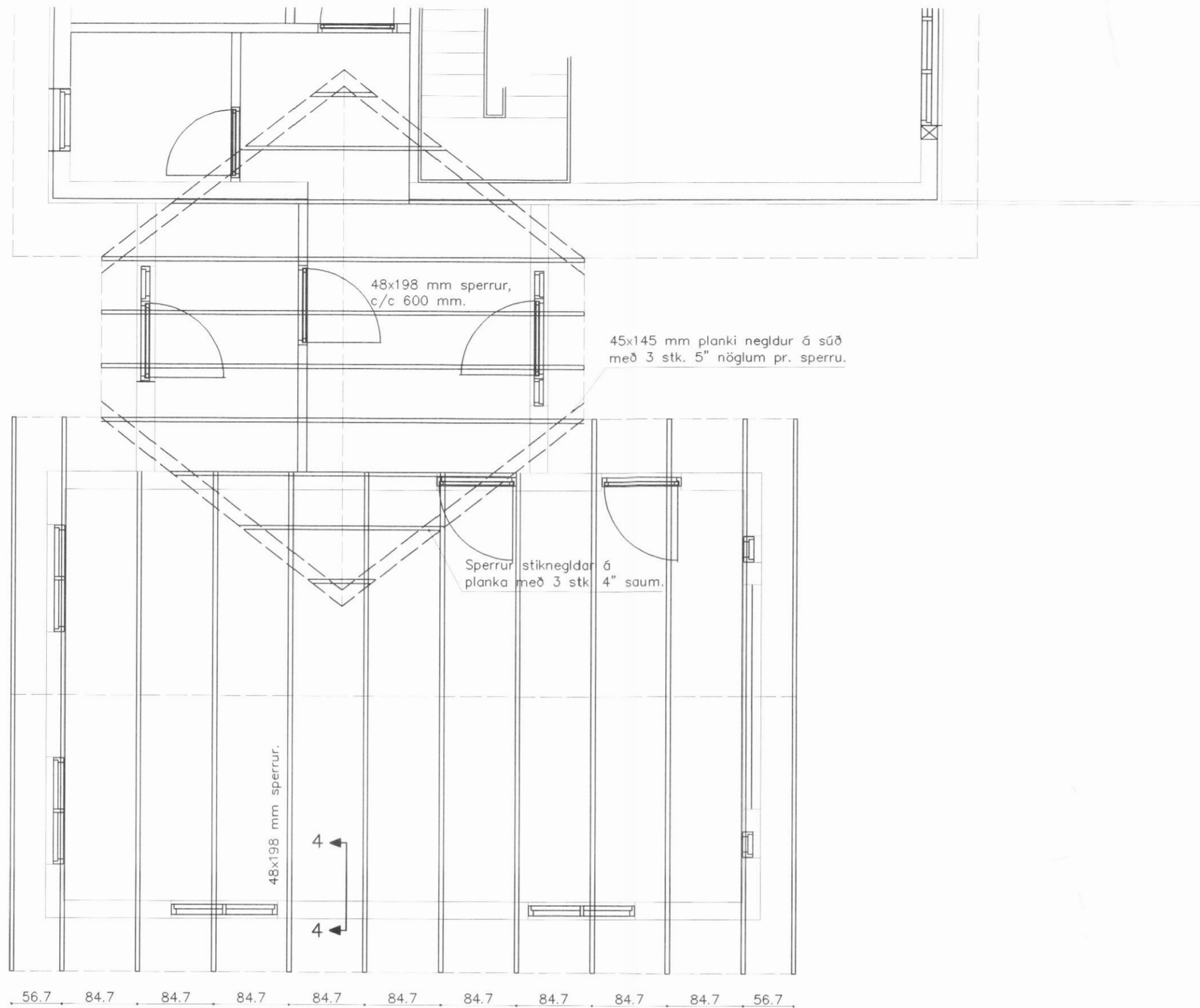
SPERRUPLAN 1:50
