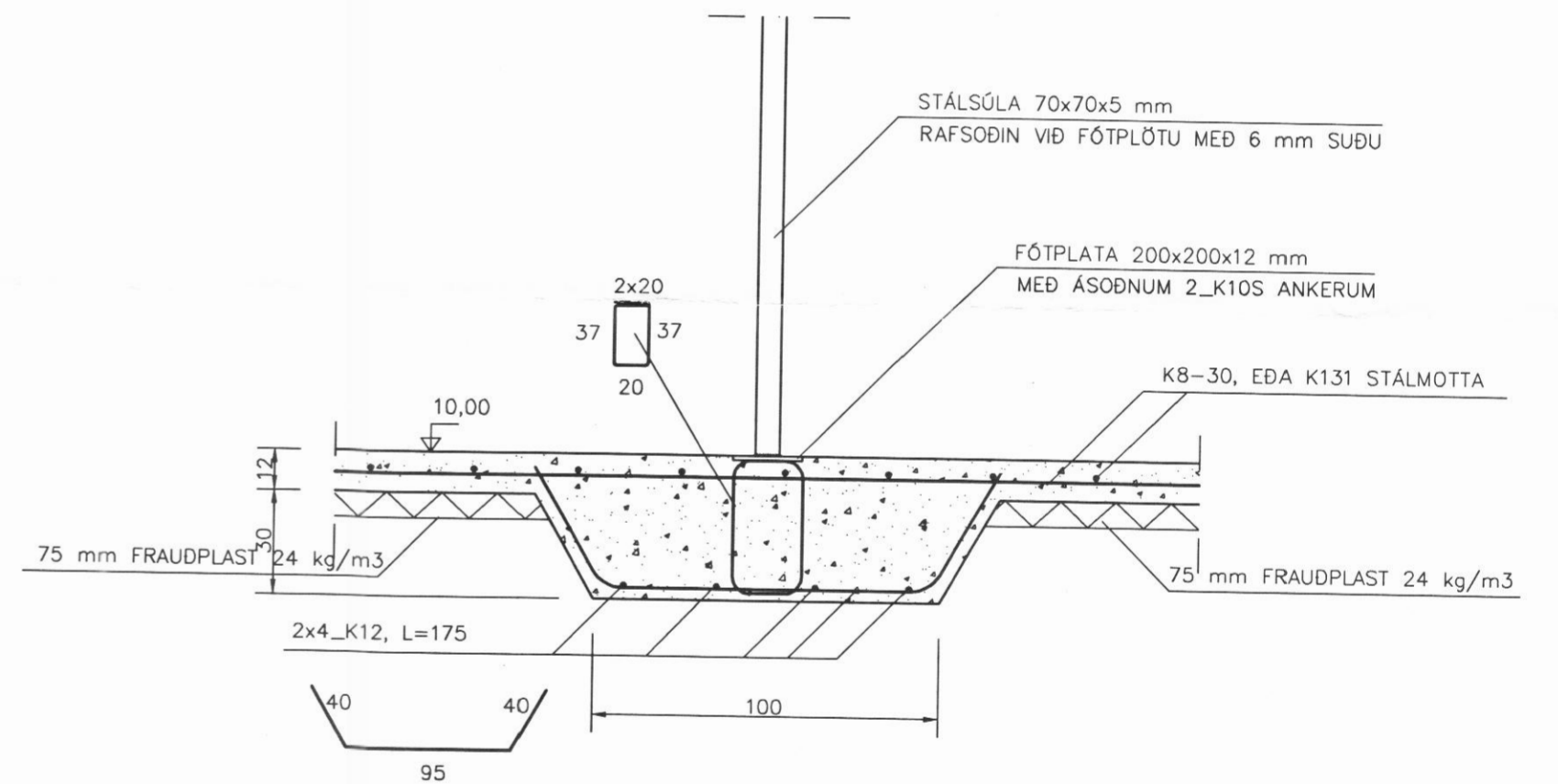
Snið 3, 1:20
