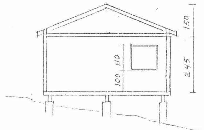
SNID A-A
