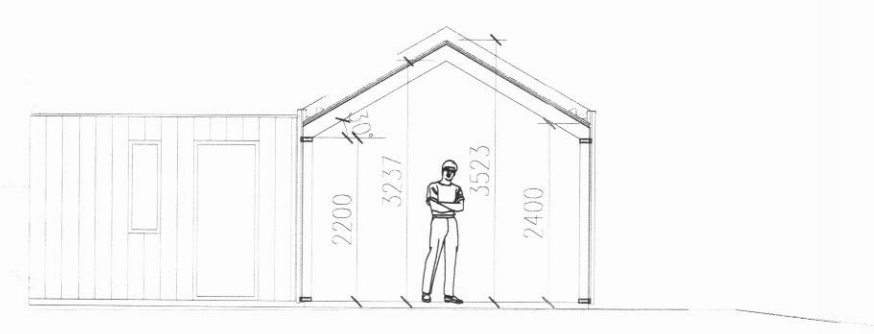
Skurður E-E
