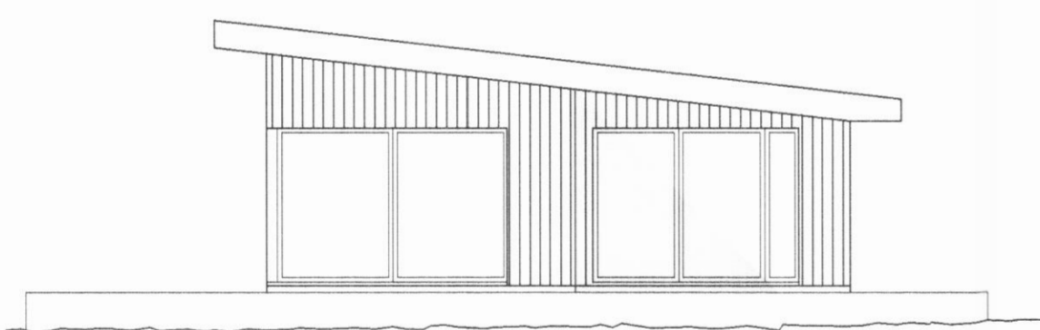
SUD-VESTUR.1:100
