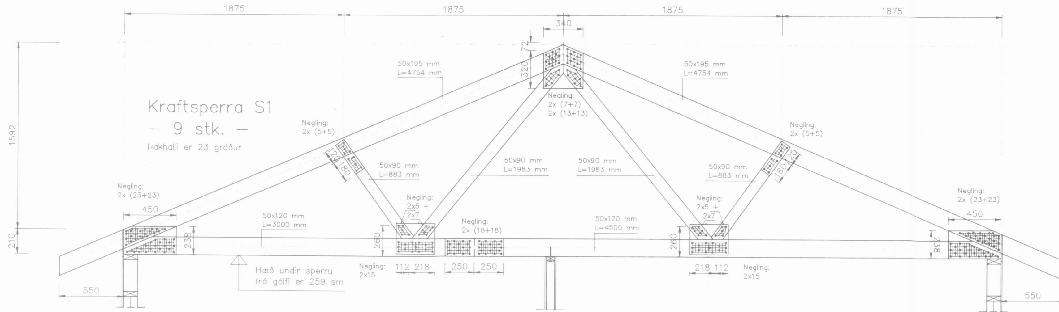
Yfirlitsmynd kraftsperru 1:20
