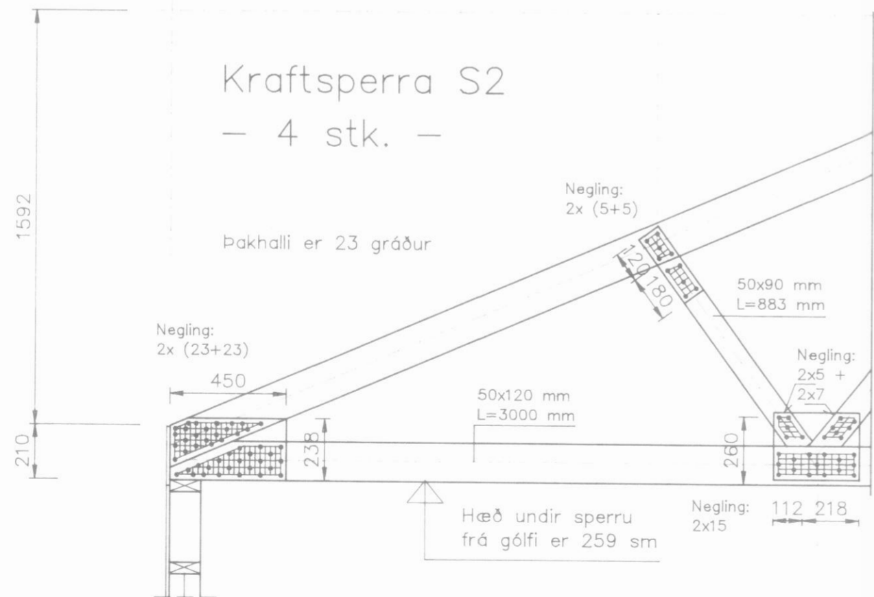
Yfirlitsmynd kraftsperru 1:20
