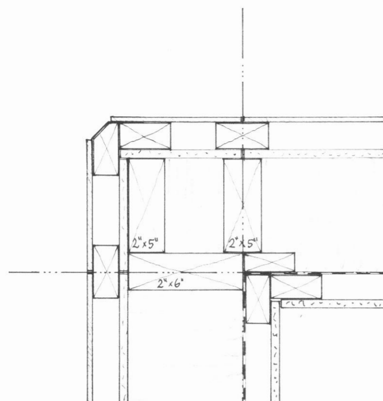
HLUTI A 1:5
