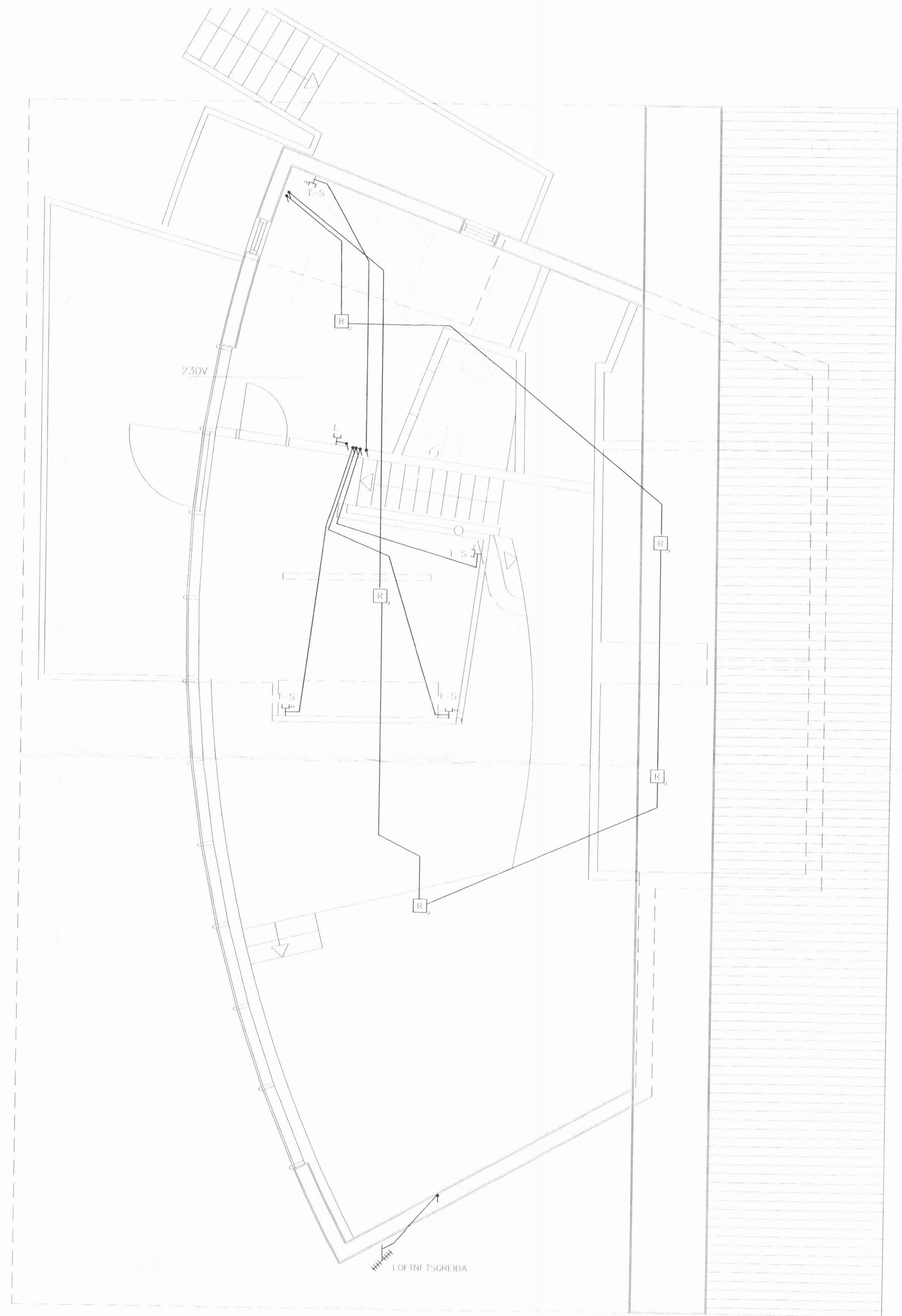
GRUNNMYND 3. HÆÐ 1:50
