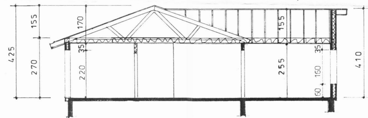
SNÍÐ B-B M; 1:100
