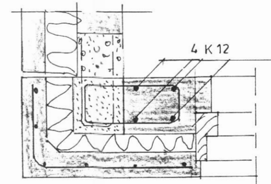
SNÍÐ A-A M; 1:10 Í EINIÐGU V9
