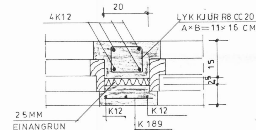
SNÍÐ D-D M; 1:10 Í EINIÐGU V1
