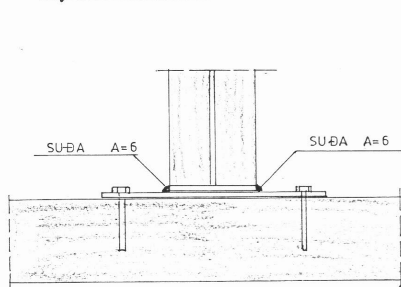
FESTING INNVEGGJAR VIÐ GÓLF LÖÐRETT SNÍÐ M; 1:5
