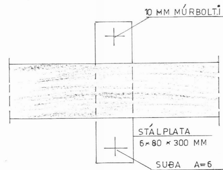
FESTING INNVEGGJAR VIÐ GÓLF LÁGRÉTT SNÍÐ M; 1:5
