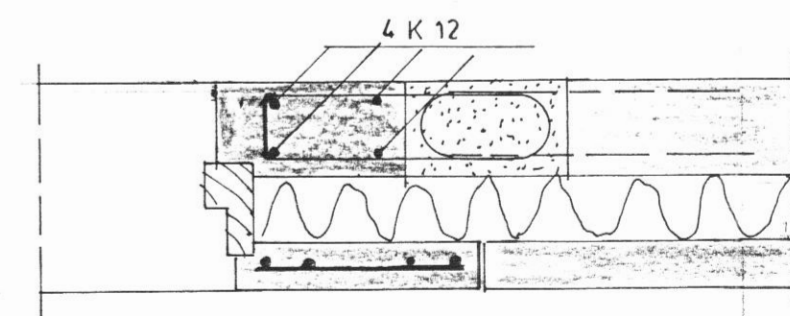
SNÍÐ B-B M; 1:10 Í EINIÐGU V9
