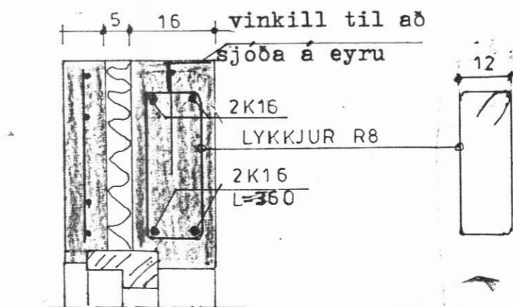
SNÍÐ C-C M; 1:10 Í EINIÐGU V11
