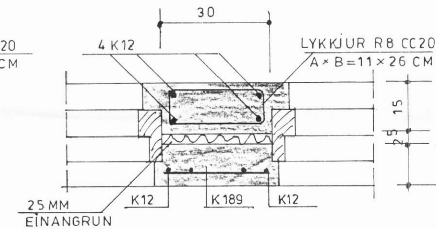
SNÍÐ E-E M; 1:10 Í EINIÐGU V8
