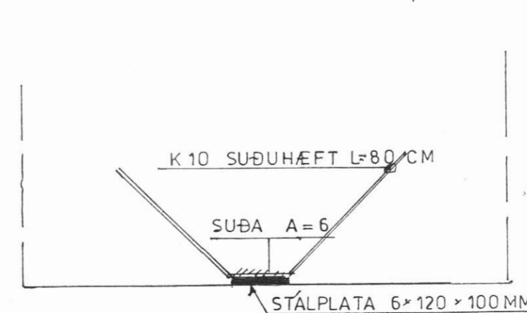
INNSTEYPT PLATA Í INNVEGG TIL FESTINGAR VIÐ GÓLF
