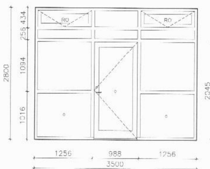
GLUGGI NR. G-16/H-12
