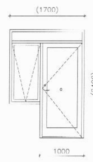
HURÐ NR. H-14
