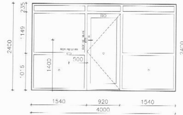
GLUGGI NR. G-12/H-10
