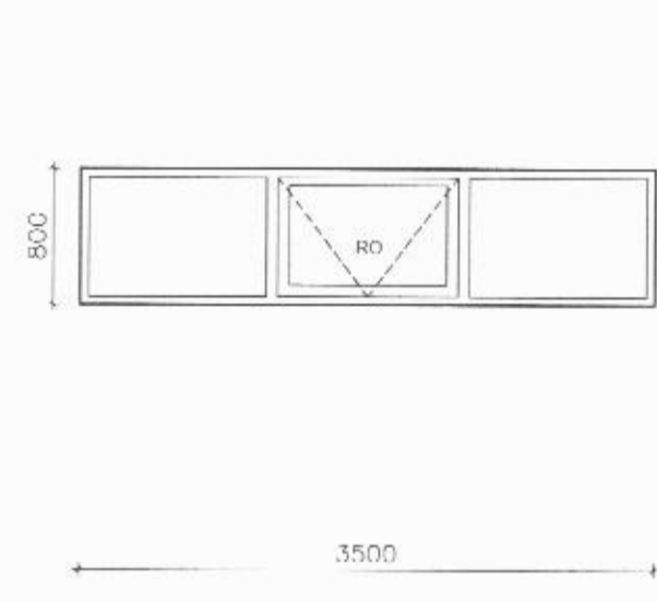
GLUGGI NR. G-17
