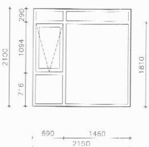
GLUGGI NR. G-14 A
