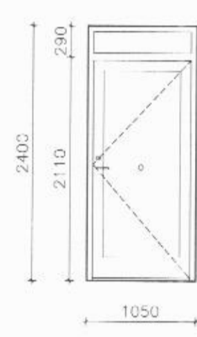
HURÐ NR. H-11 A
