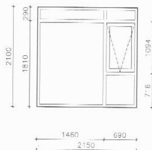
GLUGGI NR. G-14
