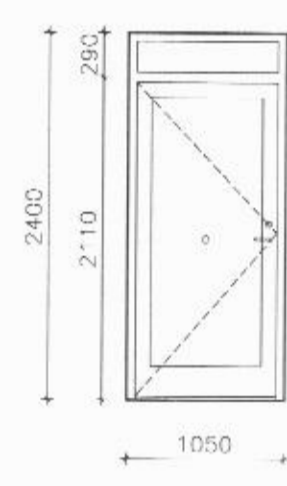
HURÐ NR. H-11
